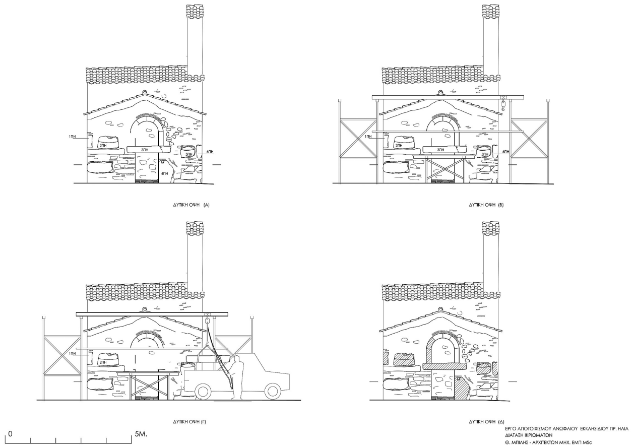
Εικ. 17. Σχέδια τοποθέτησης των ικριωμάτων και των ανυψωτικών διατάξεων στο εκκλησίδιο του Προφήτη Ηλία.
