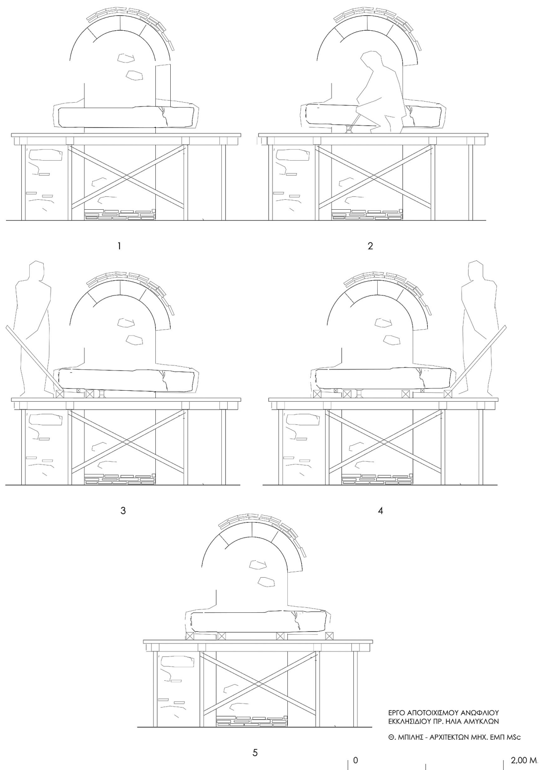
Εικ. 18. Σχέδια της διαδικασίας αποτοίχισης του ανωφλίου από το εκκλησίδιο του Προφήτη Ηλία.
