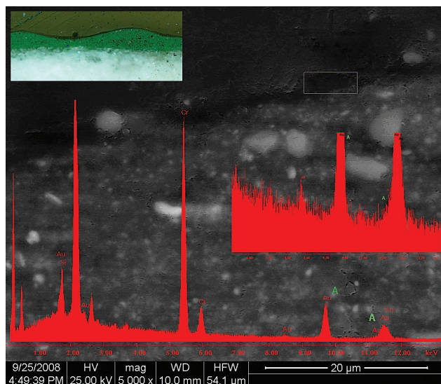
Εικ. 9. Ανάλυση μικροστροφωματογραφικής τομής SEM/EDX, όπου δεν ανιχνεύεται ο ιχνηθέτης.
