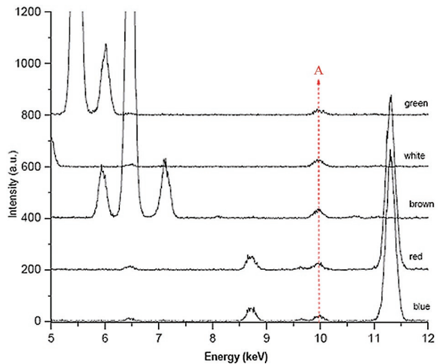
Εικ. 14. Φάσματα XRF πριν και μετά την εφαρμογή ιχνηθέτη, καθώς και μετά την αφαίρεσή του για τον έλεγχο των δυνατοτήτων αντιστροφής.
