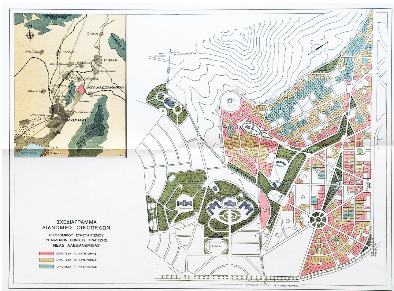
Εικ. 2. Ν. Ζουμπουλίδης, το δεύτερο πολεοδομικό σχέδιο του οικισμού, 1929. Αθήνα, Μουσείο Μπενάκη - Αρχεία Νεοελληνικής Αρχιτεκτονικής.
