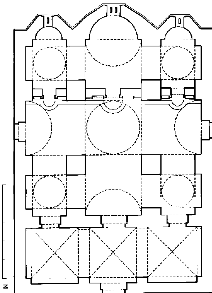
Σχ. 1. Κάτοψη
