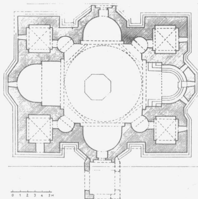
Εικ. 8. Γεωργία. Mtskheta, Ναος Dshwari. Προστώ με μονόλοβα ἀνοίγματα. Κάτοψη.
