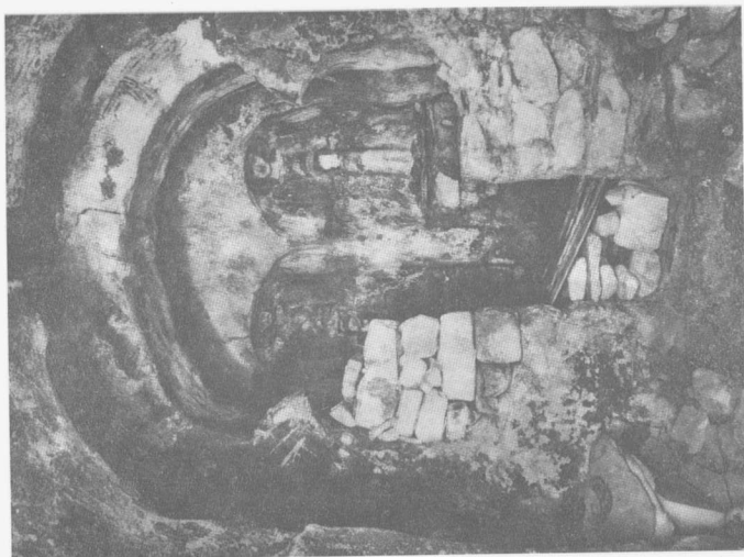
Είκ. 2. Μάνη. Ναός Ἁγ. Παντελεήμονα στοὺς Μπουλαριούς. Κατάλοιπα τοῦ κτιστοῦ τέμπλου με τῶξωτά ἀνοίγματα.
