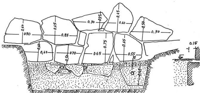
Εικ. 3. Τομή και όψη του ανατολικού τείχους του Διψηλίου με θέα προς τη Δύση.
