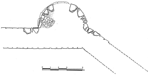
Εικ. 8. Το μεσημβρινό τείχος του Δισπηλιού στο σημείο της υλάσεως.
