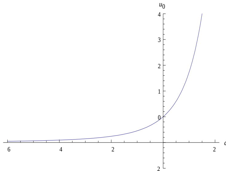
Chapter 6 Σχήμα 3.1. Η κρίσιμη τιμή της θερμοκρασίας στο πρόβλημα Stefan
