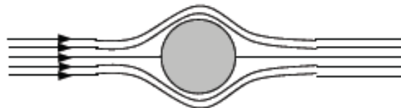
Ροή Stokes γύρω από σφαίρα ( N_{Re} \ll 1 )
