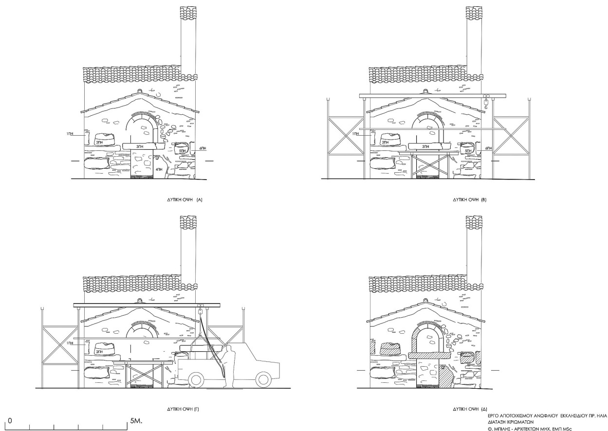
Εικ. 17. Σχέδια τοποθέτησης των κριωμάτων και των ανυψωτικών διατάξεων στο εκκλησίδιο του Προφήτη Ηλία.
