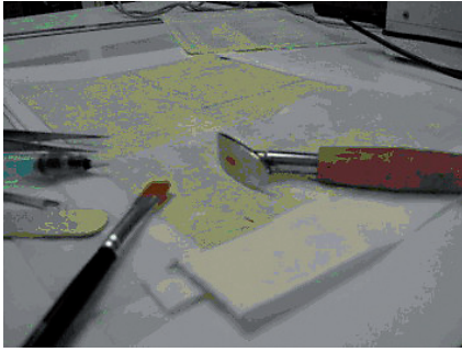
Εικ. 16. Εργασίες τοπικής ενίσχυσης αποδυναμωμένων περιοχών και επιπεδοποίηση.
