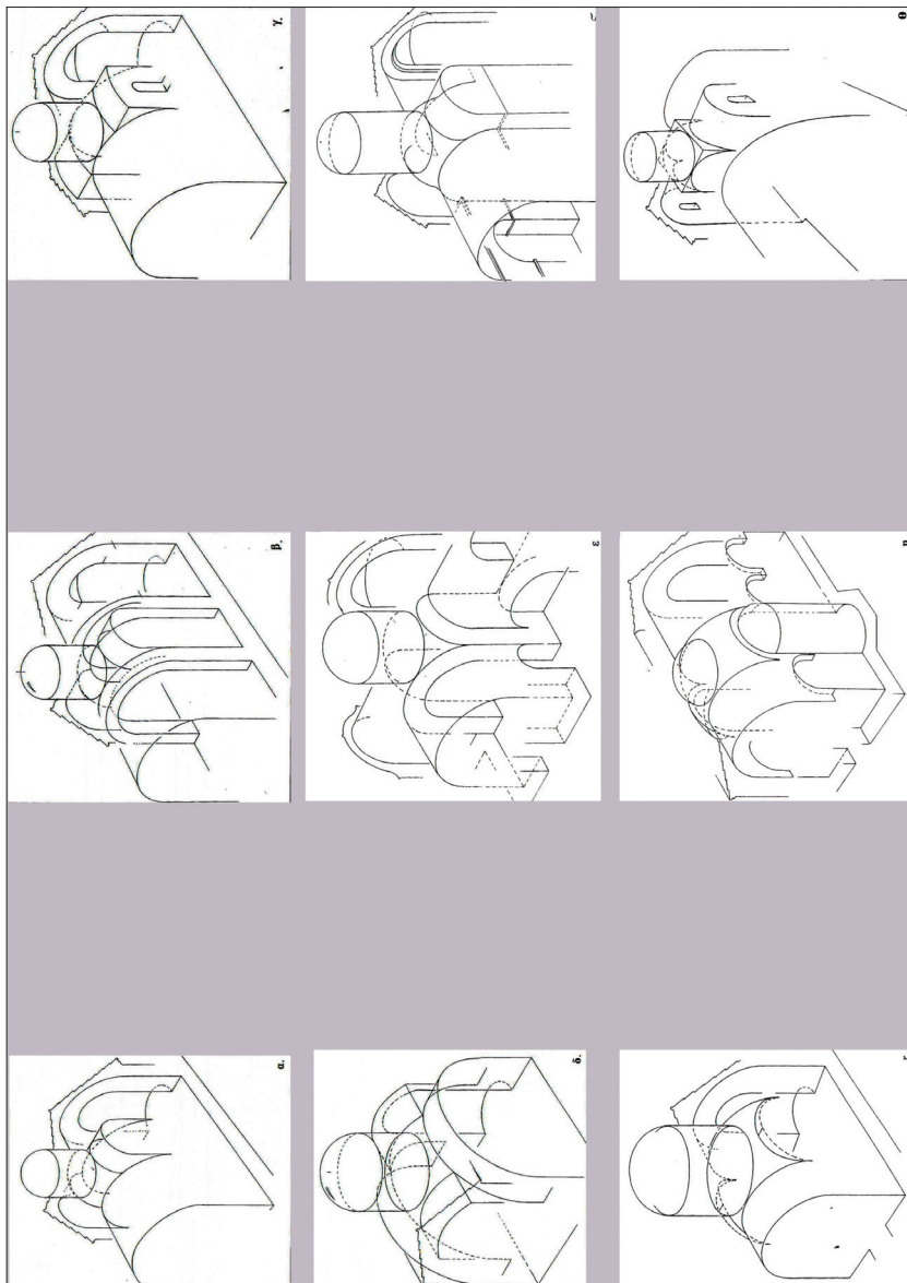
Είχ. 1. Παραλλαγές τρόπων στηρίξεως συνεπτυγμένων τρούλων κατά Χ. Μπούρα.
