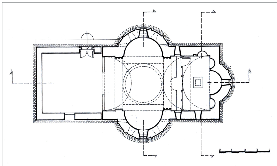
Σχέδιο 1. Κάτοψη.
