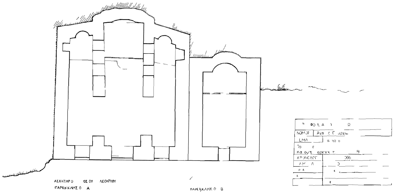
Σχέδ. 1: Κάτοψη παρεκκλησιων τοῦ ἀσκητηρίου τοῦ Ὁσίου Λεοντιου
