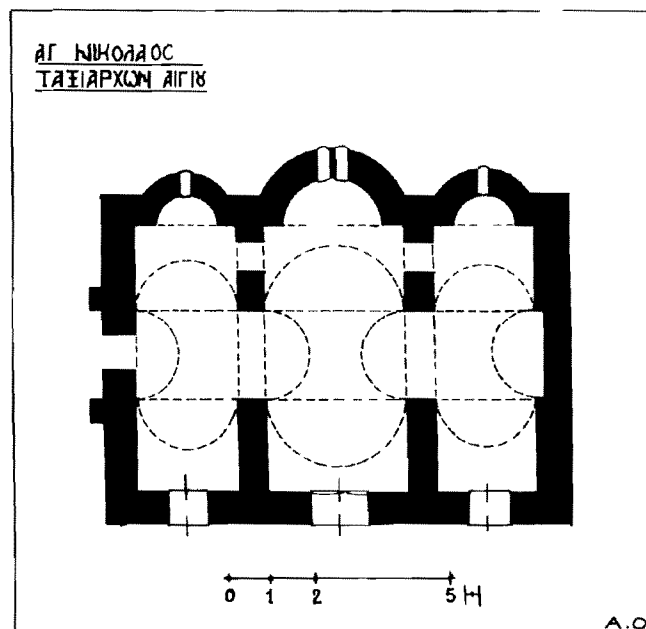
Σχέδ.5: Ναός Ἁγίου Νικολάου. Κάτοψη Ἁ. Ὁρλάνδου.
