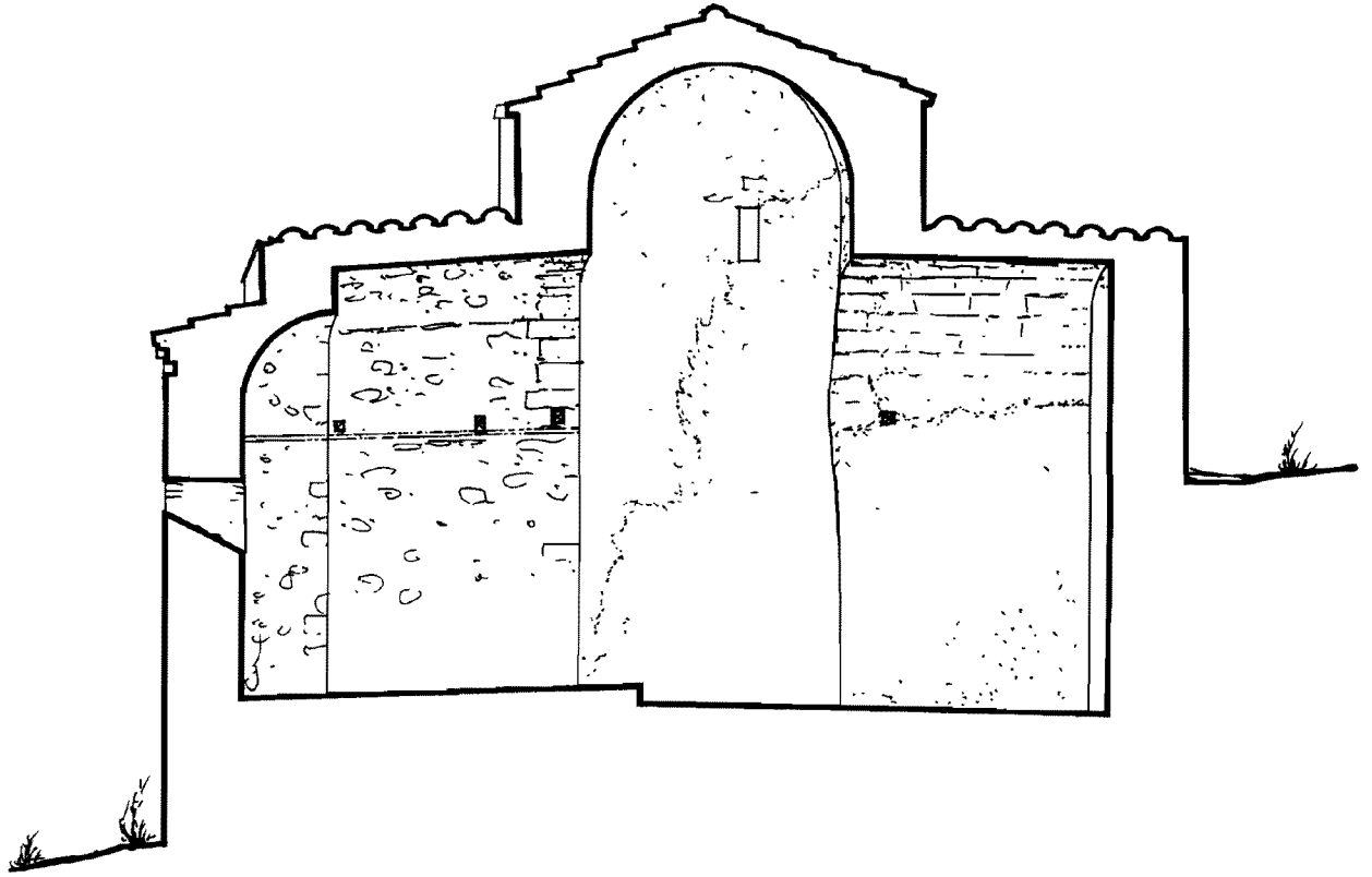
Σχέδ. 16: Ναός του Ἁγίου Νικολάου. Ἀνατολική ὄψη. Τάφος 1.
