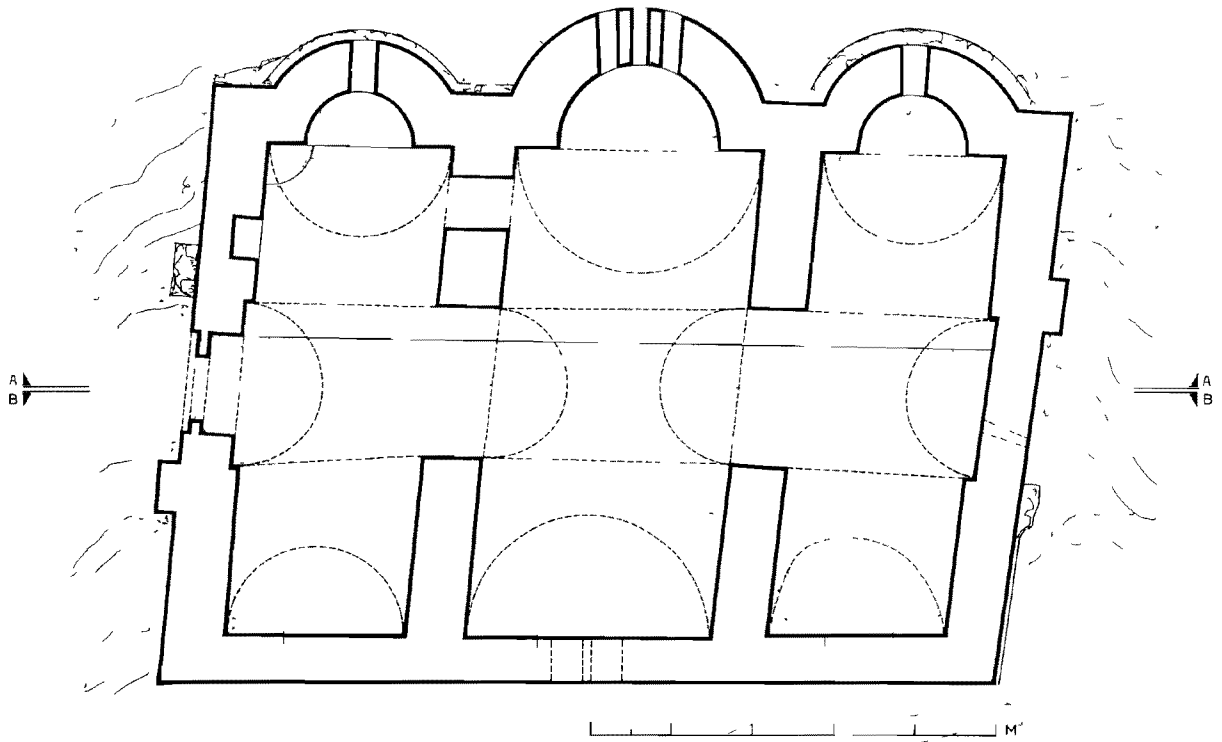
Σχέδ. 6: Ναός Ἁγίου Νικολάου. Κάτοψη Στ. Μαμαλοῦκου.
