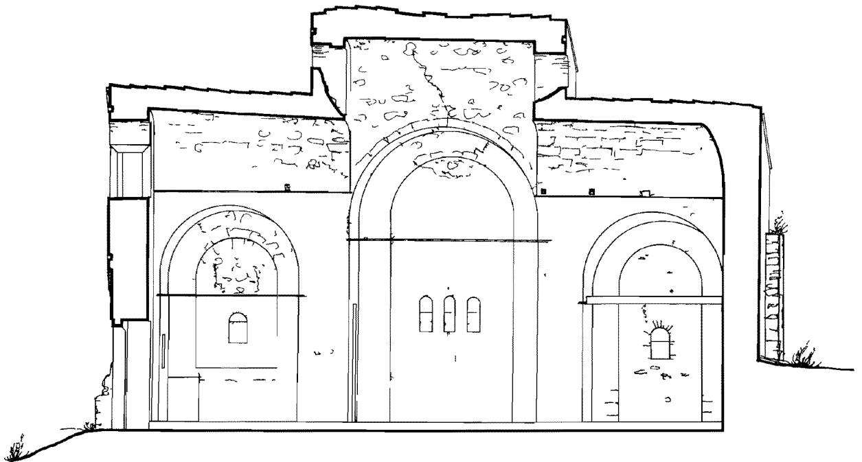
Σχέδ. 11: Ἅγιος Νικόλαος. Τομή ΑΑ.
