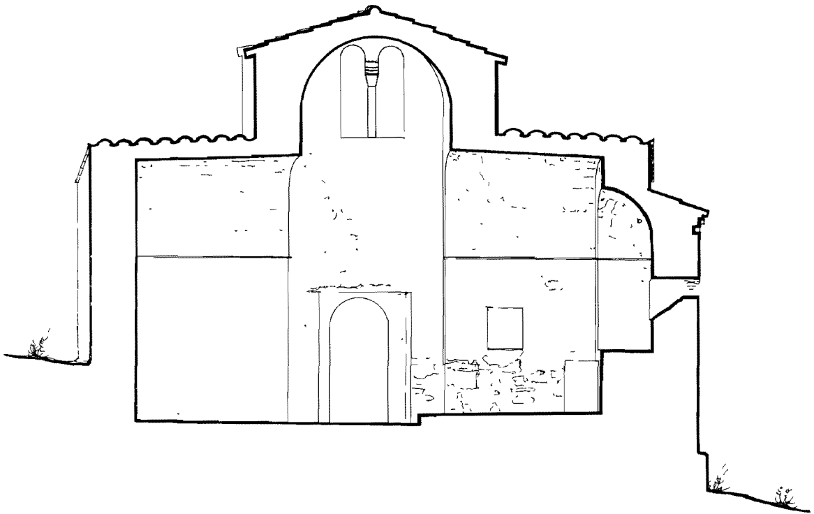
Σχέδ. 13: "Αγιος Νικόλαος. Τομή ΓΓ.
