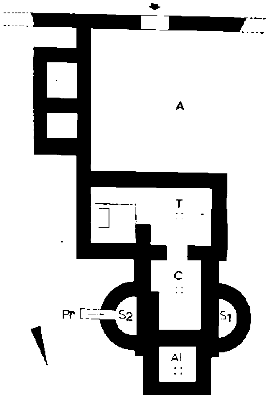
Σχ. 4. Πρωτοβυζαντινὸ λουιρὸ ὁδοῦ Γούναρη. Σχεδιαστικὴ κάτοψη ἀνασκαφῆς
