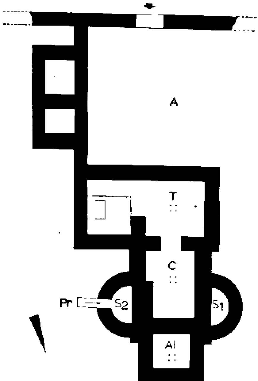
Σχ. 4. Πρωτοβυζαντινό λουτρό οδού Γούναρη. Σχεδιαστική κάτοψη ανασκαφής
