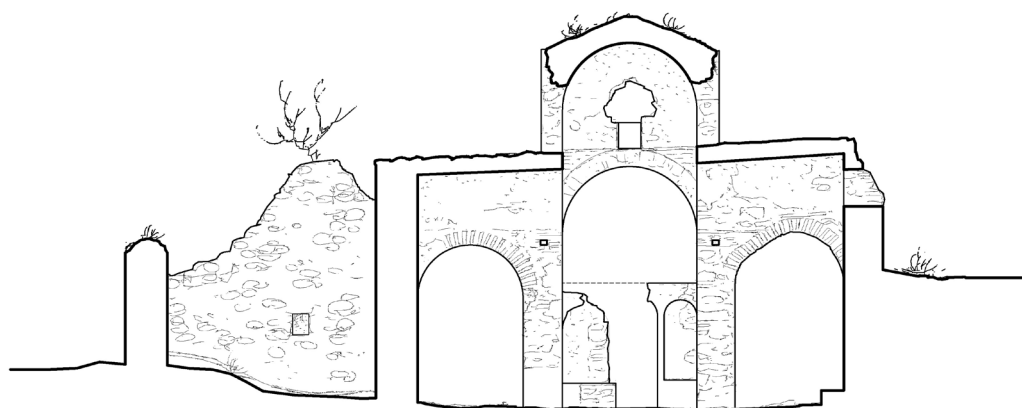
ΤΟΜΗ ΣΤ-ΣΤ
