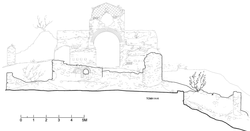
Εικ. 9. Ρέμα Σωφρόνη, Άγιος Νικόλαος, τομές κατά πλάτος.
