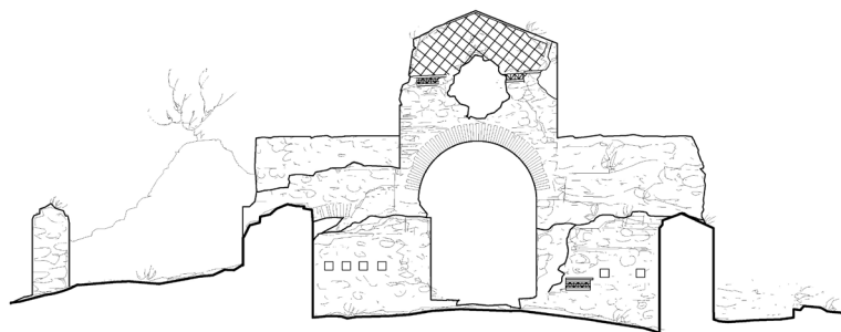
ΤΟΜΗ Ζ-Ζ
