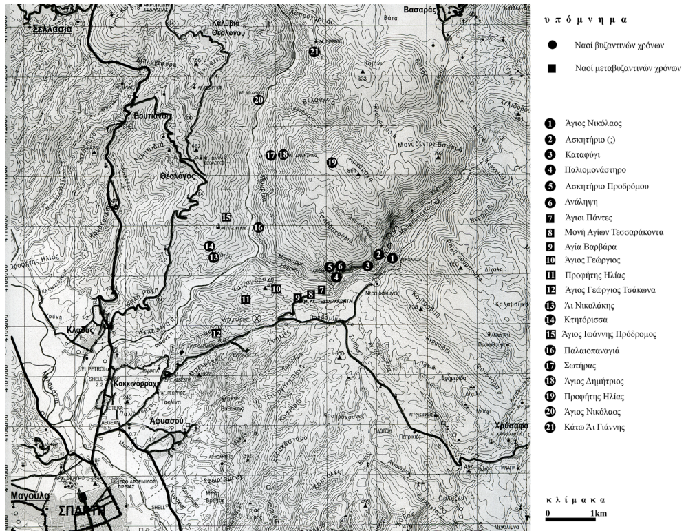
Ειχ. 1. Χάρτης της περιοχής του ρεμάτος του Σωφρόνη (Ανάβαση, Πάροννας)
