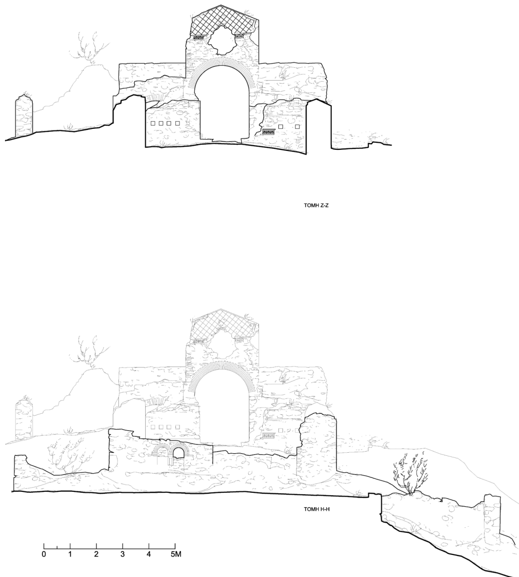
Ειχ. 9. Ρέμα Σωφρόνη, Άγιος Νικόλαος, τομές κατά πλάτος.
