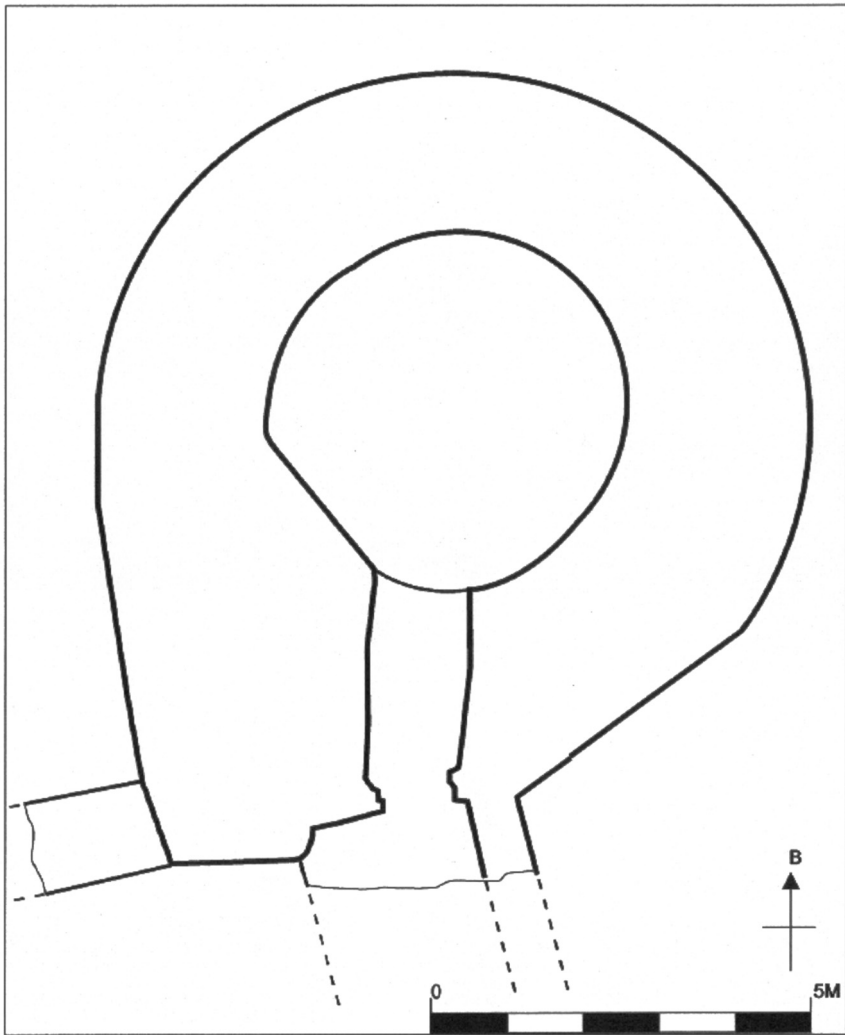
Ειχ. 14. Διδυμότειχο, Πεντάζωνο. Οριζόντια τομή στη στάθμη της εισόδου, 2012. Σχέδιο Α. ΤΣΑΝΑΚΑ.
