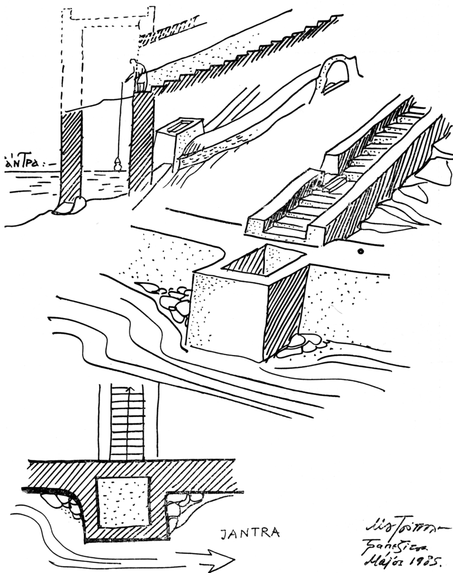
Εικ. 8. Τύρνοβο, ο πύργος του νερού. Σχεδιαστική αναπαράσταση. (MOUTSOPOULOS, Pensées et observations, σχ. 3).
