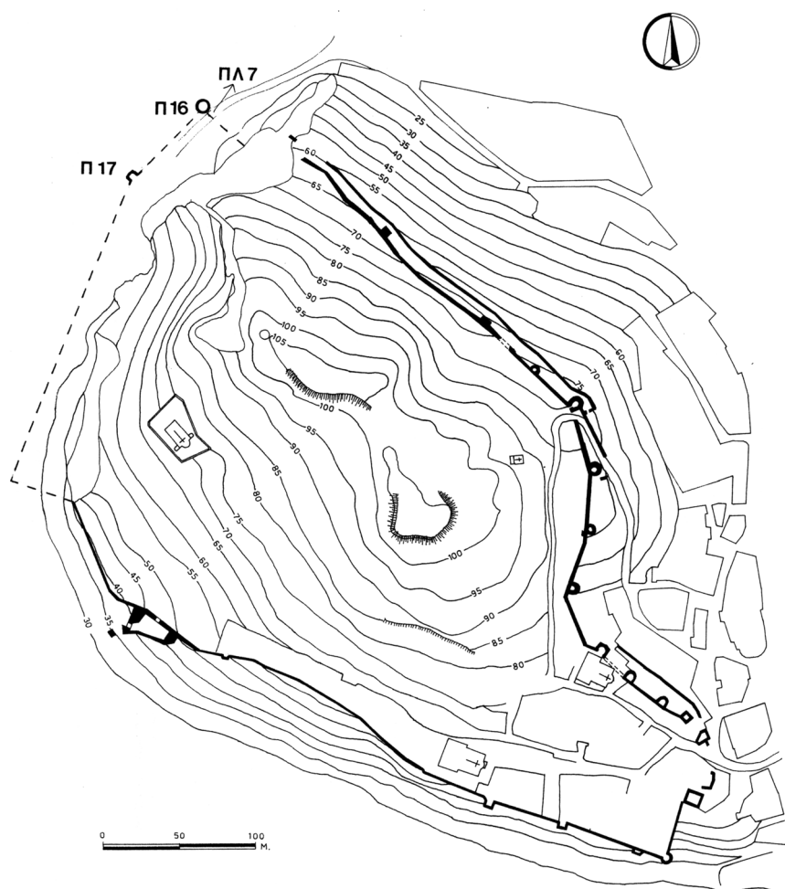
Ειγ. 1. Η οχύρωση του Διδυμοτείχου. Τοπογραφικό διάγραμμα, 1986.
