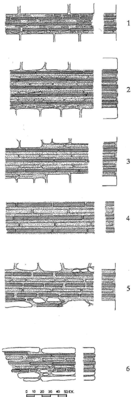
Εικ. 21. Κρυμμένη πλίνθος: 1. Φέρες, περίβολος Μονής Κοσμοσωτεΐρας. Πύργος του κωδωνοστασίου. 2. Κάστρο Διδυμοτείχου, Πεντάζωνο. 3. Πύθιο, ακρόπυργος. 4. Κως, κάστρο Παλιού Πυλίου. 5. Καβάλα, σταθμός Πετροπηγής. ΝΔ πύργος. 6. Καβάλα, ακρόπολη. Πεντάπλευρος πύργος. (ΤΣΟΥΡΗΣ - ΜΠΡΙΚΑΣ, Το φρούριο του Πυθίου , σχ. 6.)
