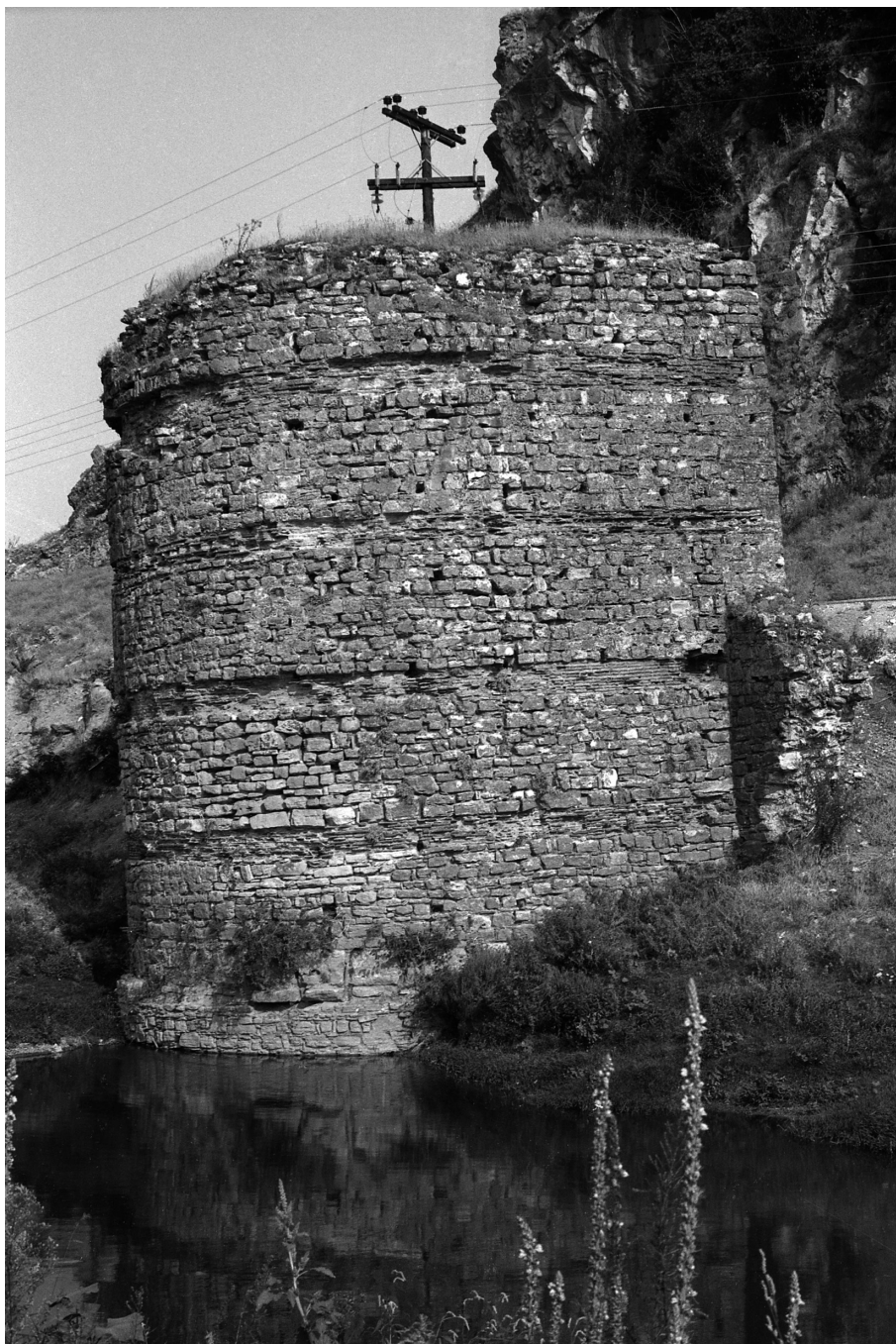
Εικ. 2. Διδυμότειχο, Πεντάζωνο. Άποψη από τα νότια. Λήψη Κ. ΤΣΟΥΡΗ, 1986. (Αρχείο 12ης ΕΒΑ).
