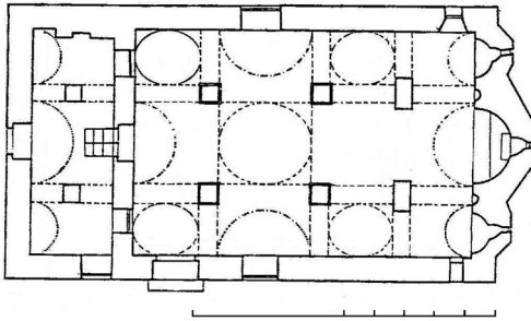
Σχ. 5. Κάτοψη Αγίου Νικολάου Καρύταινας (ΜΟΥΤΣΟΠΟΥΛΟΣ, Γορτυνία, 61, ειχ. 33)
