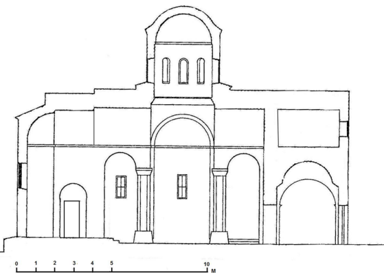
Σχ. 25. Τομή κατά μήκος καθολικού μονής Ζερμπίτσας (ΑΝΔΡΟΥΛΙΔΑΚΗ, Ζερμπίτσα, πιν. ΙΔ΄ ειχ. 10)
