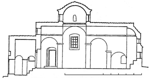
Σχ. 6. Τομή κατά μήκος Αγίου Νικολάου Καρύταινας (ΜΟΥΤΣΟΠΟΥΛΟΣ, Γορτυνία, 61, ειχ. 33)
