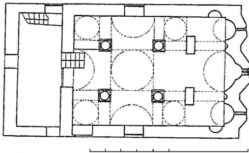
Σχ. 7. Κάτοψη Ζωοδόχου Πηγής Καρύταινας (ΜΟΥΤΣΟΠΟΥΛΟΣ, Γορτυνία, 50, ειχ. 26)
