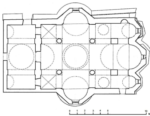
Σχ. 24. Κάτοψη καθολικού μονής Ζερμπίτσας (ΑΝΔΡΟΥΛΙΔΑΚΗ, Ζερμπίτσα, πιν. ΙΒ΄ ειχ. 6)
