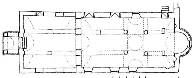
Σχ. 18. Κάτοψη Ταξιαρχών Ερμιόνης (ΠΡΟΚΟΠΙΟΥ, Ερμιόνη, 154 εικ. 3)
