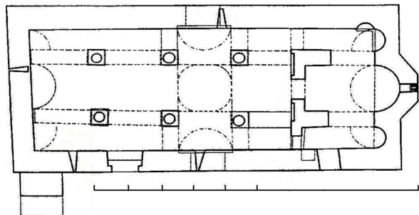
Σχ. 17. Κάτοψη Κοίμησης Θεοτόκου στο Λυγουριό (ΑΣΛΑΝΙΔΗΣ - ΠΙΝΑΣΗ, Λυγουριό, 14, εικ. 2)
