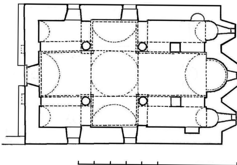
Σχ. 15. Κάτοψη καθολικού μονής Παλαιοπαναγίας Κυνουρίας (ΣΤΟΥΦΗ- ΠΟΥΛΗΜΕΝΟΥ, Παλαιοπαναγία Κυνουρίας, 194, εικ. 2)
