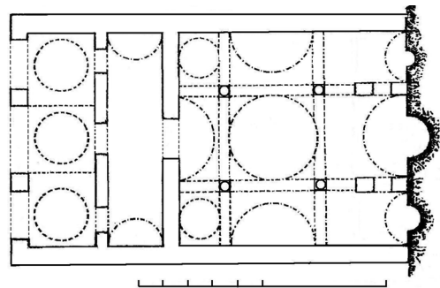
Σχ. 16. Κάτοψη καθολικού μονής Μεγάλου Σπηλαίου (ΣΩΤΗΡΙΟΥ, Μεγάλο Σπήλαιο, 50 εικ. 5)
