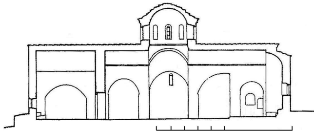
Σχ. 14. ΤΟΜΗ ΚΑΤΑ ΜΗΚΟΣ ΑΓΙΟΥ ΔΗΜΗΤΡΙΟΥ ΣΤΑ ΧΡΥΣΑΦΑ (ΧΡΥΣΟΥΛΑΚΗ- ΣΠΑΝΟΥ, ΚΑΡΥΩΤΟΥ, Άγιος Δημήτριος στα Χρύσαφα Λακωνίας, 289, ΕΙΚ. 6)
