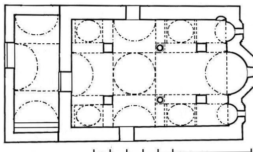
Σχ. 8. Κάτοψη καθολικού Αγίου Νικολάου Βαρσών (ανασχεδίαση βάσει του : ΜΟΥΤΣΟΠΟΥΛΟΣ, Αί παρὰ τήν Τρίπολιν μοναί, 422, εικ. 22)
