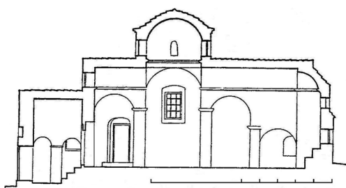
Σχ. 6. Τομή κατά μήκος Αγίου Νικολάου Καρύταινας (ΜΟΥΤΣΟΠΟΥΛΟΣ, Γορτυνία, 61, εικ. 33)
