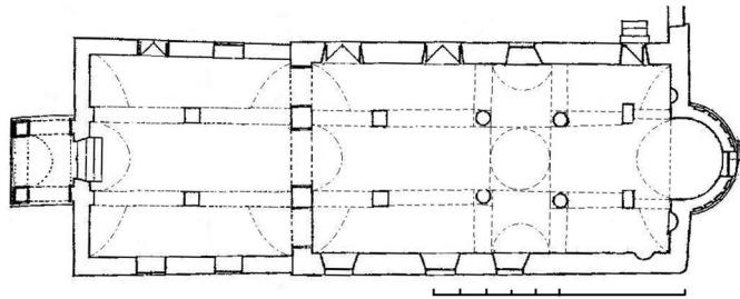
Σχ. 18. Κάτοψη Ταξιαρχών Ερμιόνης (ΠΡΟΚΟΠΙΟΥ, Ερμιόνη, 154 ειχ. 3)
