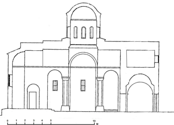
Σχ. 25. Τομή κατά μήκος καθολικού μονής Ζερμίτσας (ΑΝΔΡΟΥΛΙΔΑΚΗ, Ζερμίτσα, πιν. ΙΔ΄ ειχ. 10)
