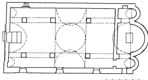
Σχ. 20. Κάτοψη Αγίου Νικολάου Λικινίου Μονεμβασιάς (Χ. ΚΑΛΛΙΓΑ, Ο Ναός του Αγίου Νικολάου του Λικινίου στη Μονεμβασία, Εκκλησίες 7, Θεσσαλονίκη 2013, 58 ειχ. 2)
