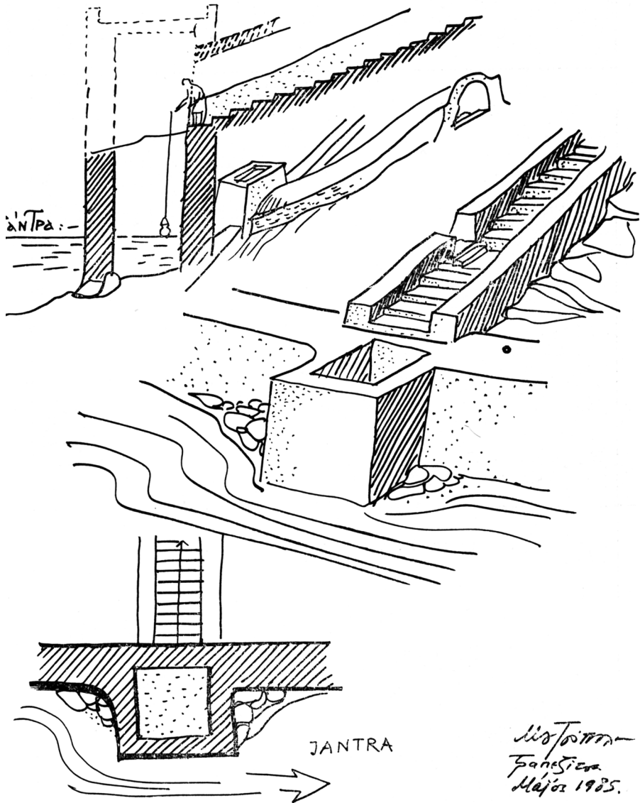
Ειχ. 8. Τύρνοβο, ο πύργος του νερού. Σχεδιαστική αναπαράσταση. (MOUTSOPOULOS, Pensées et observations, σχ. 3).
