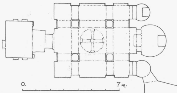
Είκ. 11. Καππαδοκία. Matchan. παρεκκλήσιο Bezir Khanе. Κάτοψη, τρούλλος με νευρώσεις που σχηματίζουν σταυρό.
