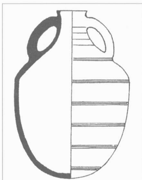
Εικ. 5. Σχέδιο καὶ φωτογραφία ὑστερορωμαϊκῶν/πρωτοβυζαντινῶν ἀμφορέων 2 καὶ 13 (LRA 2, LRA 13).
