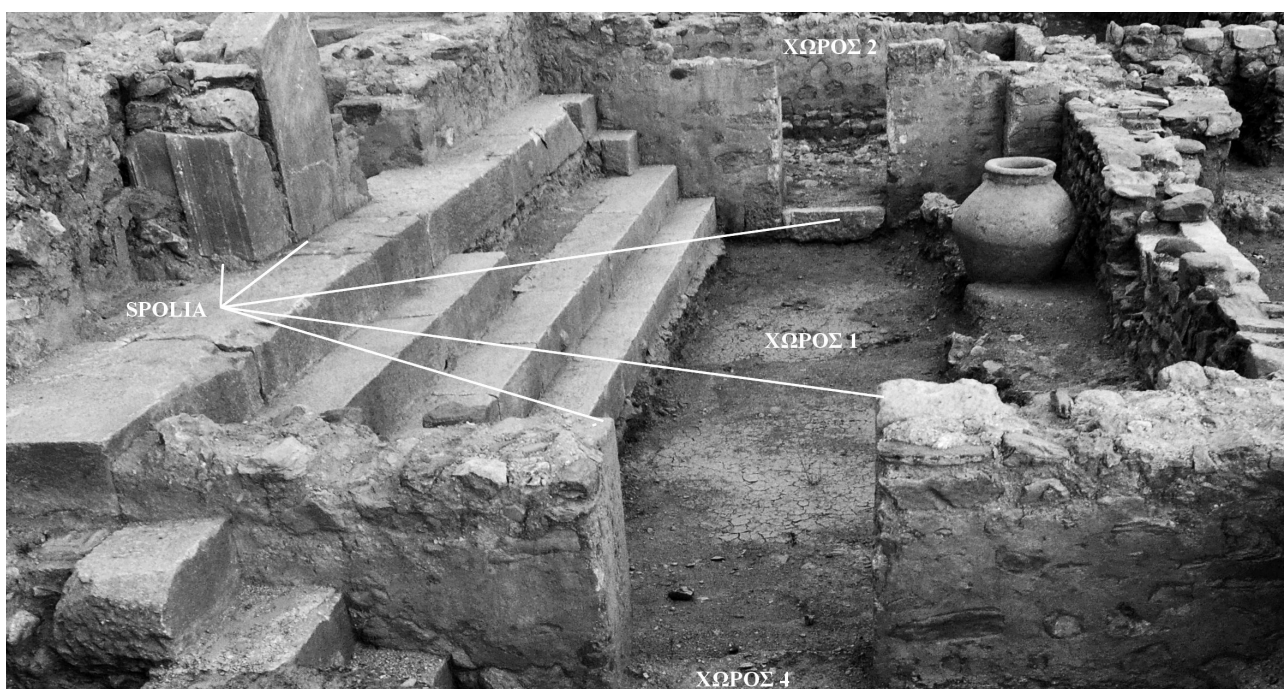
Εικ. 4. Βόρειος Τομέας. Τριμερές οικοδόμημα, εσωτερικό. Άποψη από βόρεια.
