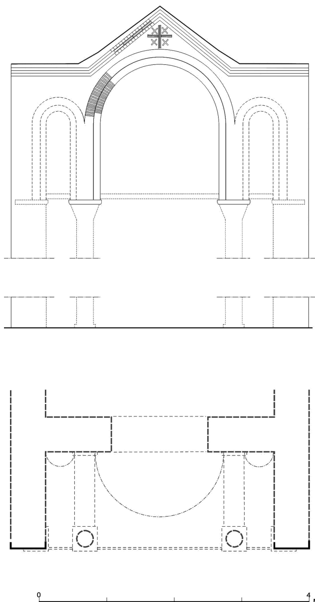
Εικ. 4. Θεσσαλονίκη. Ο βυζαντινός τοίχος (πυλώνας) της αφήγησης του Ντίνου Χριστιανόπουλου. Σχεδιαστική απόδοση όψης και κάτοψης.
