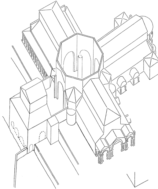
Fig. 44. Kastron de Christophoros, construit dans la partie occidentale du bras ouest du martyron cruciforme, axonométrie.
