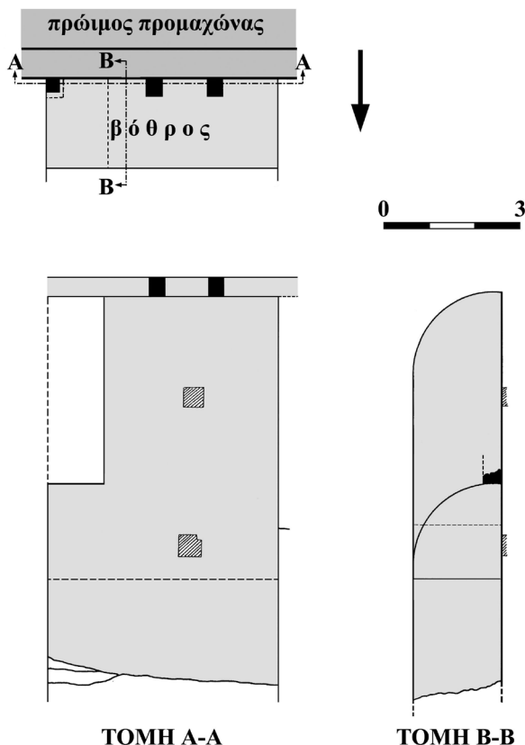
Εικ. 3. Ρόδος. Προμαχώνας Αγίου Γεωργίου. Κάτοψη και τομή του του βόθρου.
