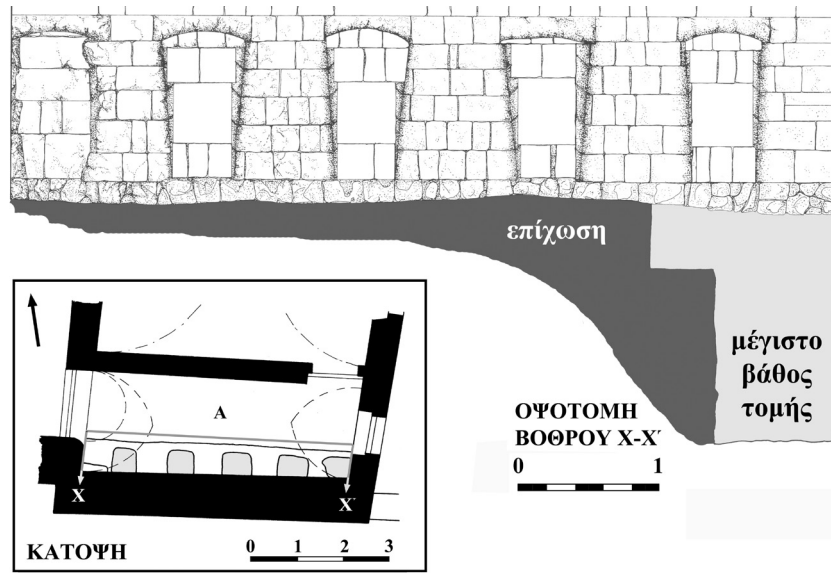
Εικ. 6. Ρόδος. Κτήριο Villaragut. Κάτοψη του αποχωρητηρίου και οψοτομή του βόθρου της Ιπποτοκρατίας.
