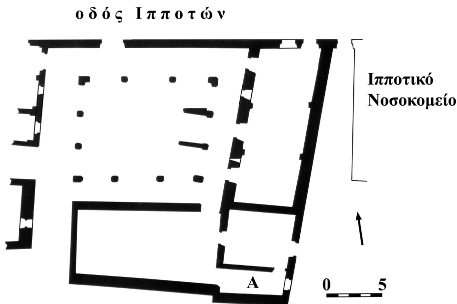
Εικ. 5. Ρόδος, Κτήριο Villaragut. Κάτοψη.
