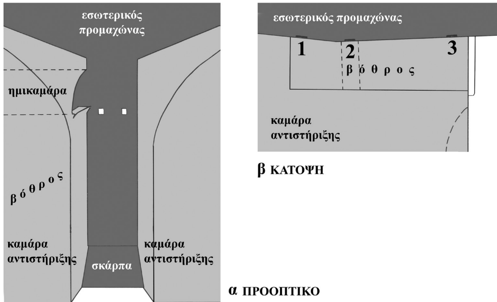
Εικ. 4. Ρόδος. Φρούριο του Αγίου Νικολάου. Προοπτικό σκαρίφημα (α) της ένταξης του βόθρου και (β) κάτοψη του δαπέδου του αποχωρητηρίου.
