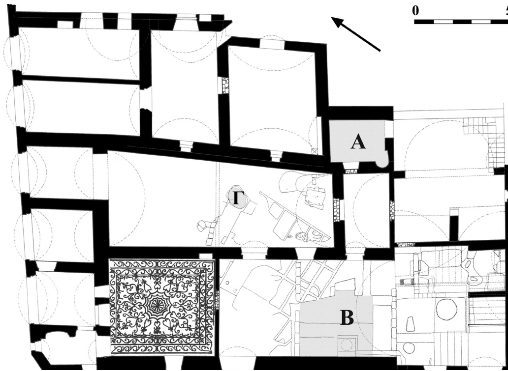
Εικ. 7. Ρόδος. Ξενώνας Αγίας Αικατερίνης. Κάτοψη ισογείου.
