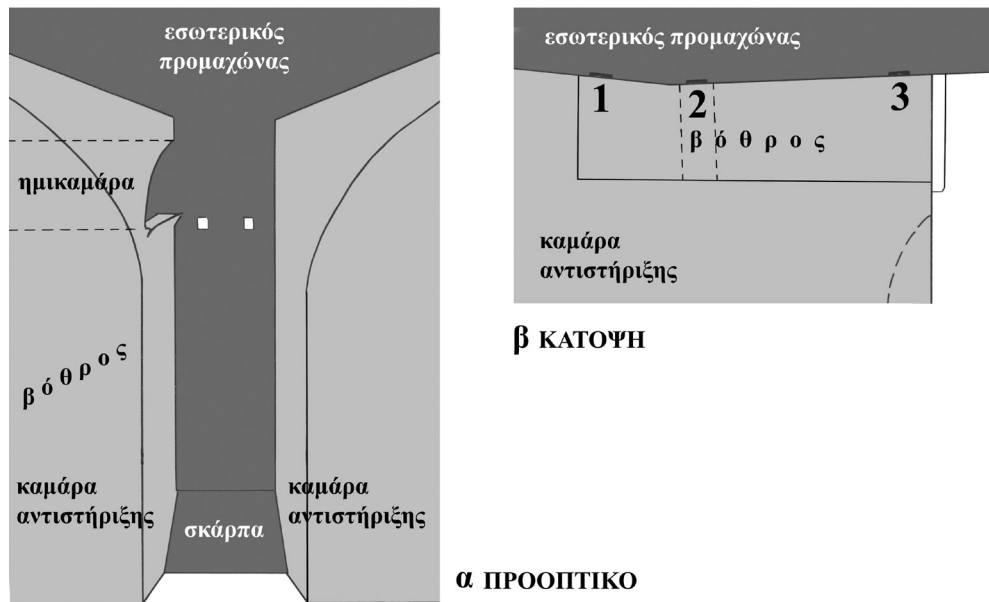
Εικ. 4. Ρόδος. Φρούριο του Αγίου Νικολάου. Προοπτικό σκαρίφωμα (α) της ένταξης του βόθρου και (β) κάτοψη του δαπέδου του αποχωρητηρίου.
