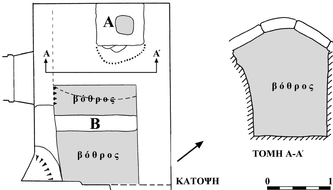
Εικ. 8. Ρόδος. Ξενώνας Αγίας Αικατερίνης. Κάτοψη και τομή αποχωρητηρίου.
