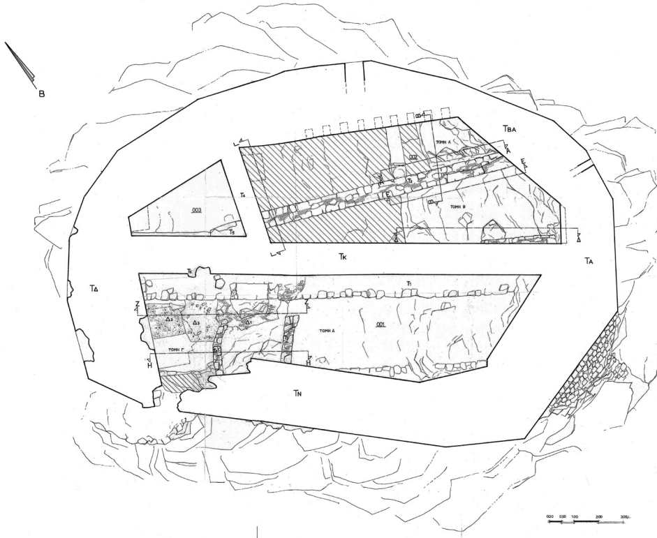
Εικ. 7. Χίος, Πιτυός. Ο πύργος. Αποτύπωση των χώρων του ισόγειου μετά την ανασκαφή.
