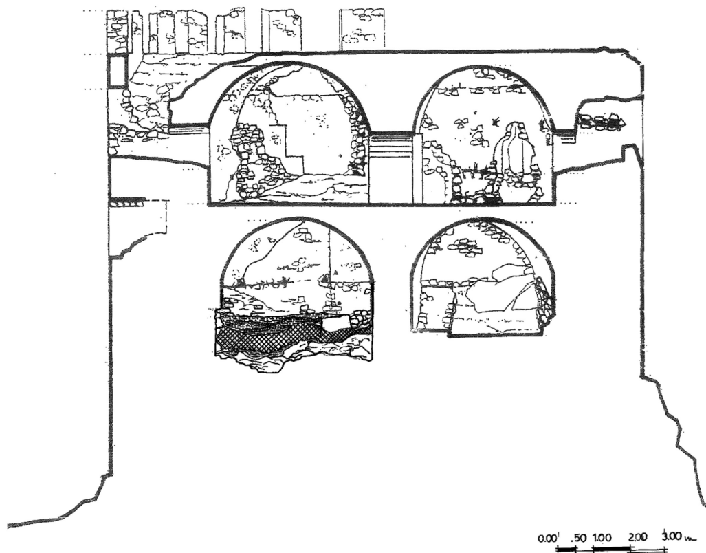
Εικ. 2. Χίος, Πιτύς. Ο πύργος. Τομή κατά πλάτος.
