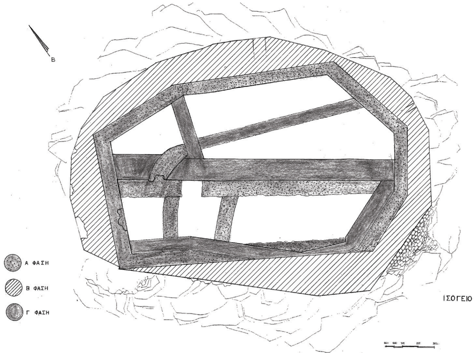
Εικ. 8. Χίος, Πιτυός. Ο πύργος. Οι τρεις οικοδομικές φάσεις του ισόγειου.
