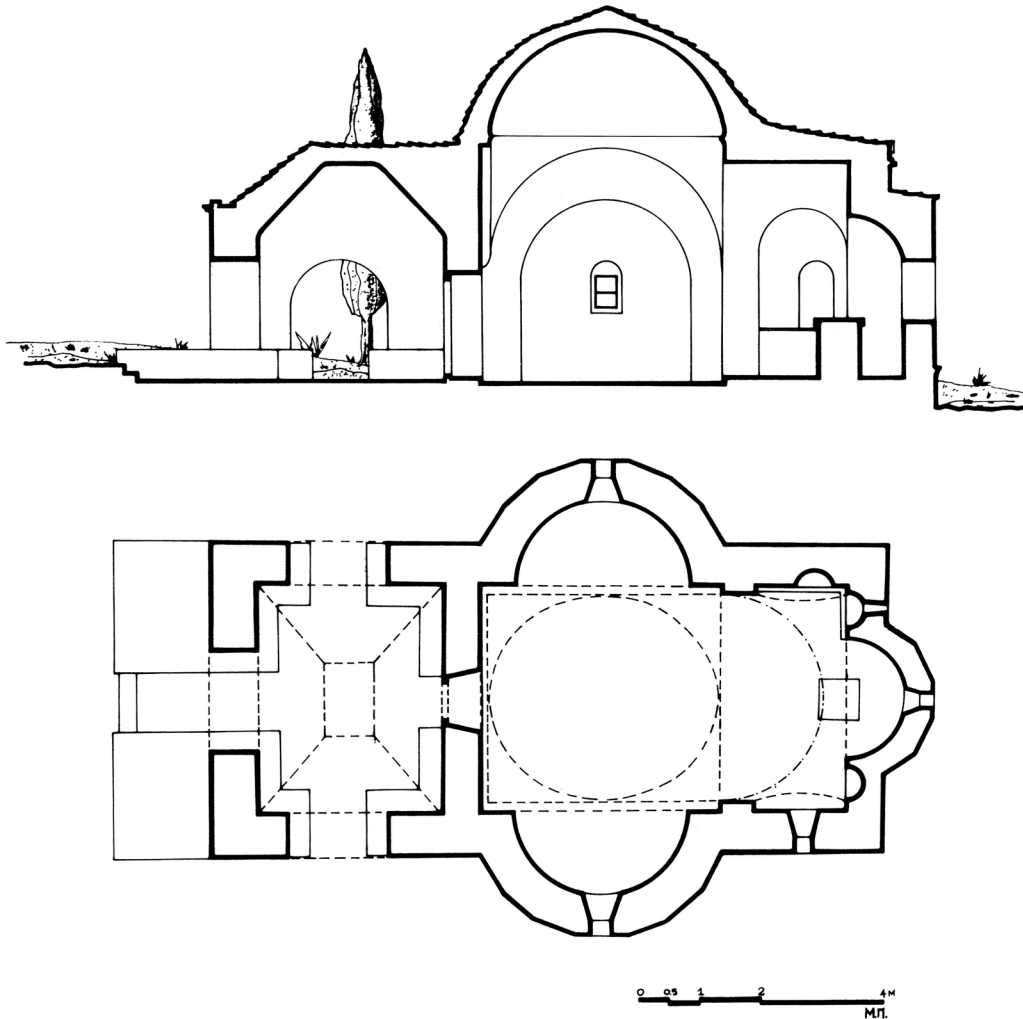
Εικ. 3. Πρασούδα. Παναγία. Κάτοψη και κατά μήκος τομή.
