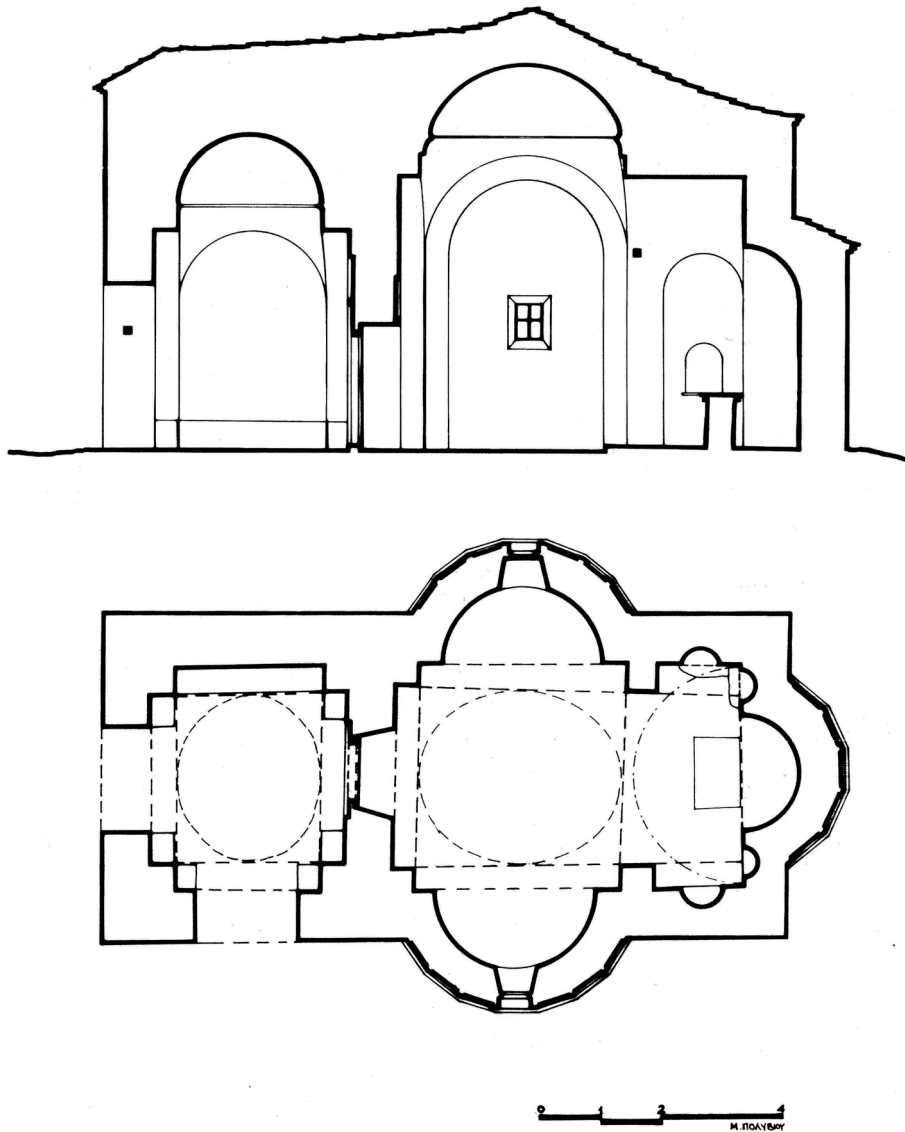
Εικ. 1. Μηλιές. Άγιος Νικόλαος ο Γέρος. Κάτοψη και κατά μήκος τομή.
