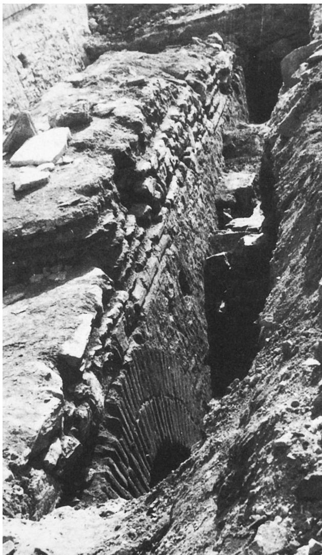
Εικ. 10. Τμήμα τοιχοποιίας της επισκοπικής βασιλικής.
