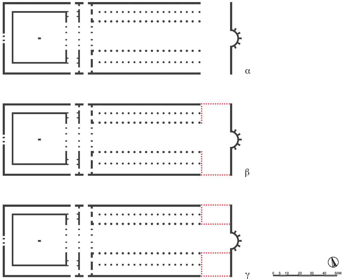
Εικ. 14. Πεντάκλιτη επισκοπική βασιλική: (α) σχεδιαστική αποκατάσταση του επιβεβαιωμένου τμήματος της κάτοψης, (β) πρόταση υποθετικής αποκατάστασης της κάτοψης ως πεντάκλιτης βασιλικής με εγκάρσιο κλίτος τύπου Α, (γ) πρόταση υποθετικής αποκατάστασης της κάτοψης ως πεντάκλιτης βασιλικής με εγκάρσιο κλίτος τύπου Β.
