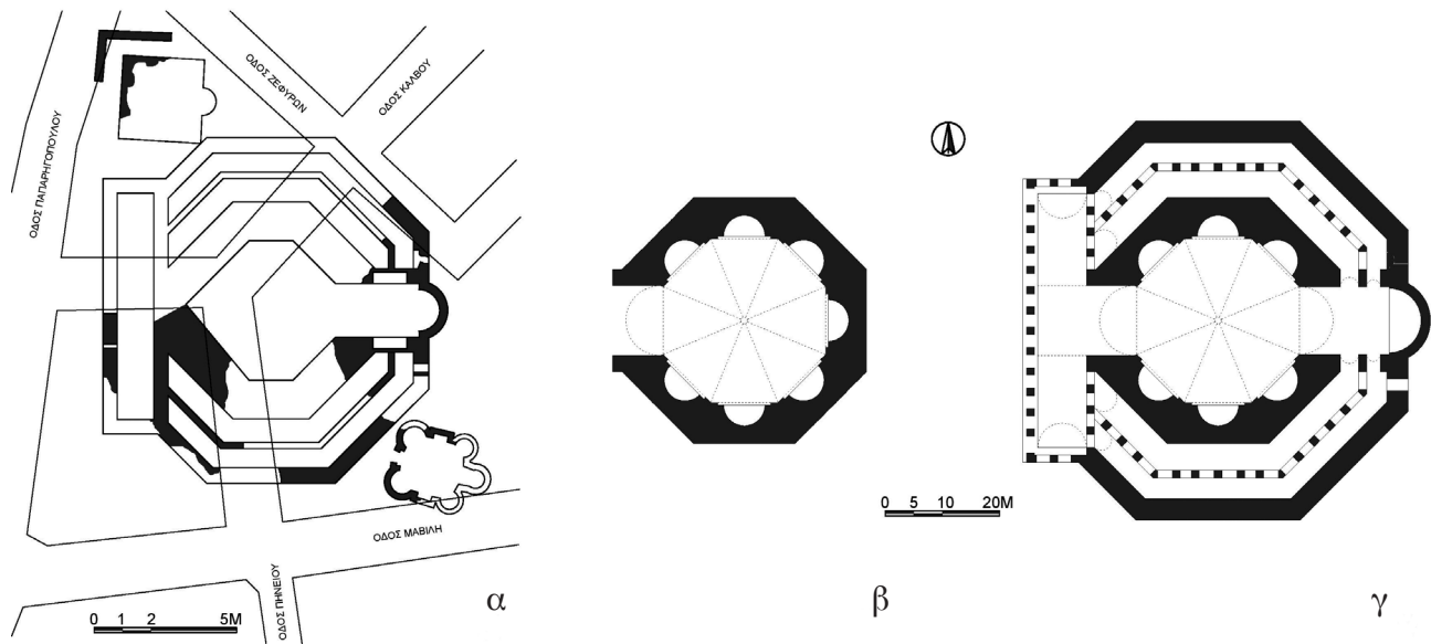
Εικ. 2. Οκτάγωνο παρά τη Χρυσή Πύλη. Κάτοψη: (α) τοπογραφικό διάγραμμα με τα ανεσκαμμένα τμήματα του αρχιτεκτονικού συγκροτήματος, (β) πρόταση υποθετικής αποκατάστασης του κτηρίου ως απλού Οκταγώνου (α' φάση – περ. 400), (γ) πρόταση υποθετικής αποκατάστασης του κτηρίου ως σύνθετου Οκταγώνου (β' φάση – περ. 500).
