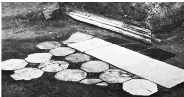
Εικ. 9. Τμήμα τοιχοβάτη και μαρμαροθέτημα από το δάπεδο του προεσβυτερίου της επισκοπικής βασιλικής.
