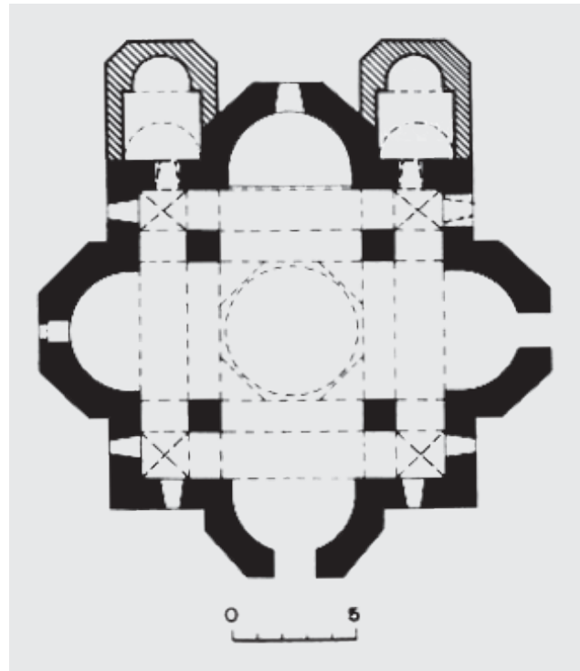
Εἰκ. 3. Ἀρμενία, Bagaran, ναὸς τοῦ Ἁγίου Ἰωάννου (624-631). Κάτοψη.
