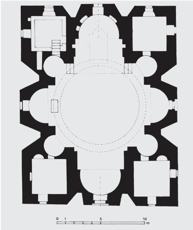
Εἰκ. 5. Ἀρμενία, Valaršapat (Etchmiadzin), ναὸς τῆς Ἁγίας Ριψιμίας (616/17, 628). Κάτοψη.
