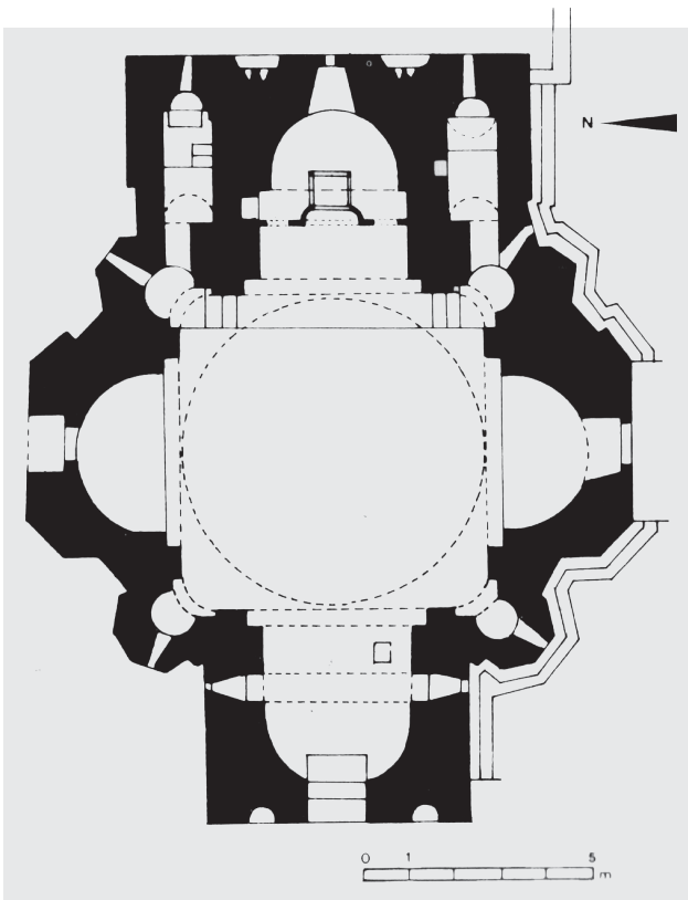
Εἰκ. 8. Τουρκία, λίμνη Van, ναὸς τοῦ Τιμίου Σταυροῦ, Agh'tamar (915-921). Κάτοψη.
