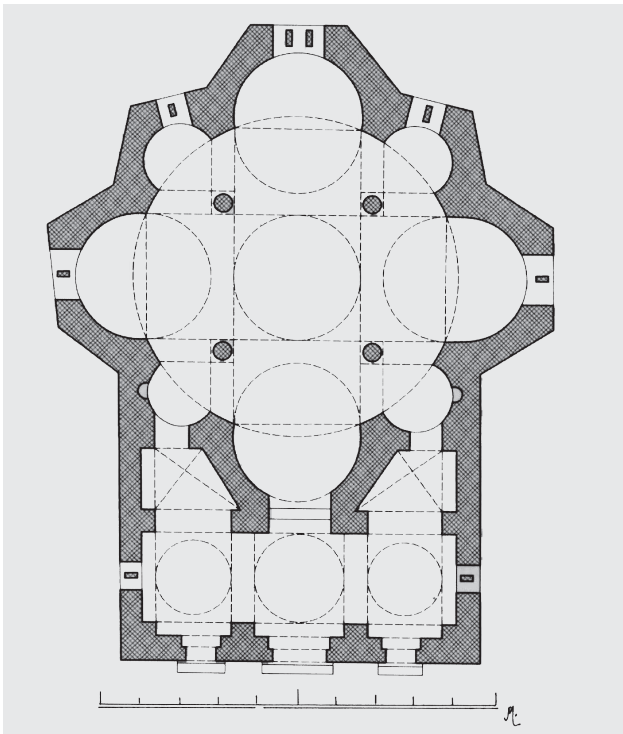
Εἰκ. 2. Ἀθήνα, ναὸς τῶν Ἁγίων Ἀποστόλων Σολάκη (π. 1000). Κάτοψη.
