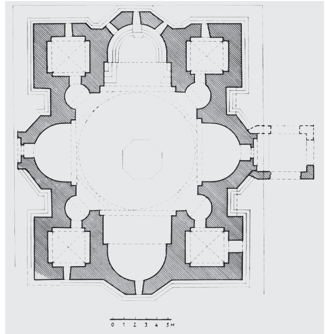
Εἰκ. 6. Γεωργία, Mtskheta, ναὸς Džvari (586-604/7). Κάτοψη.
