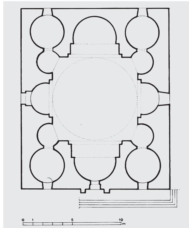
Εἰκ. 4. Ἀρμενία, καθεδρικὸς ναὸς τοῦ Avan (590). Κάτοψη.
