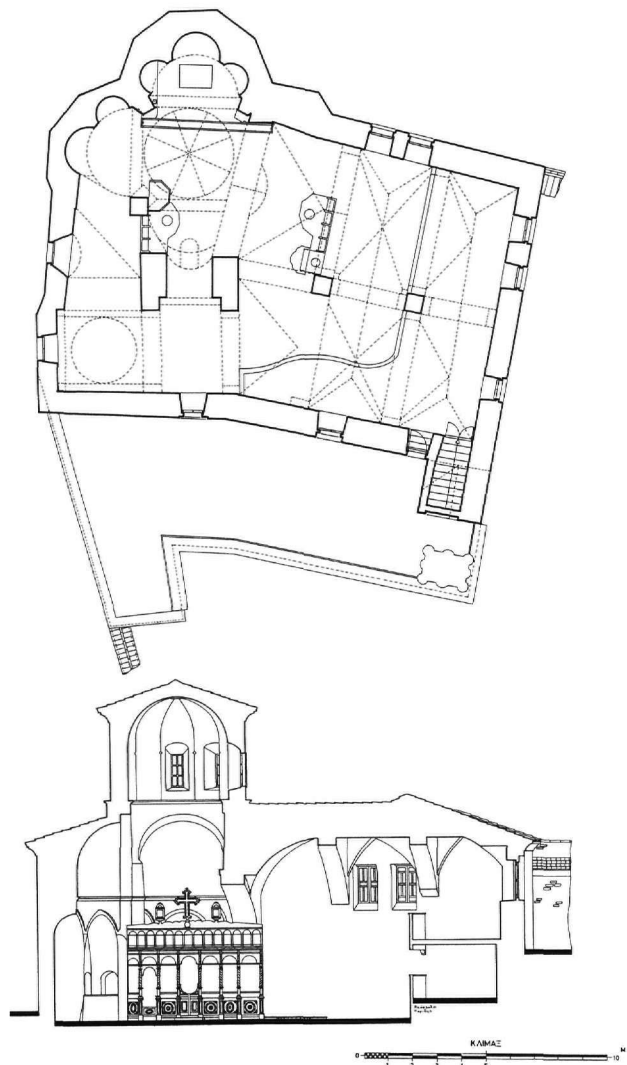
Είκ. 4. Παναγία τοῦ Μουχλίου. Κάτοψη στό ὕψος τοῦ γυναικωνίτη καί κατά πλάτος τομή. Ὑφισταμένη κατάσταση (σχέδ. Ἀ. Πορίδη).
