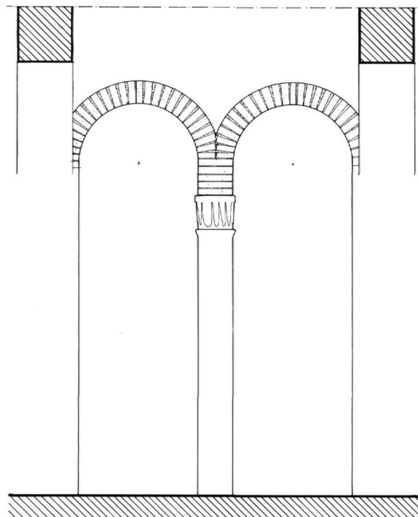
Εικ. 3. Η δίβηλη είσοδος στον κυρίως ναό.
