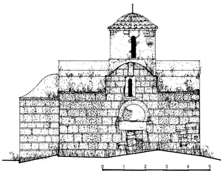
Εικ. 5. Η βόρεια όψη του ναού.
