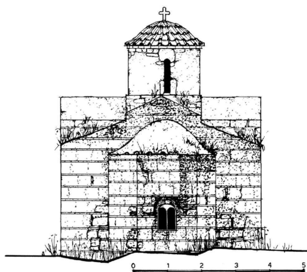
Εικ. 6. Η ανατολική όψη του ναού.
