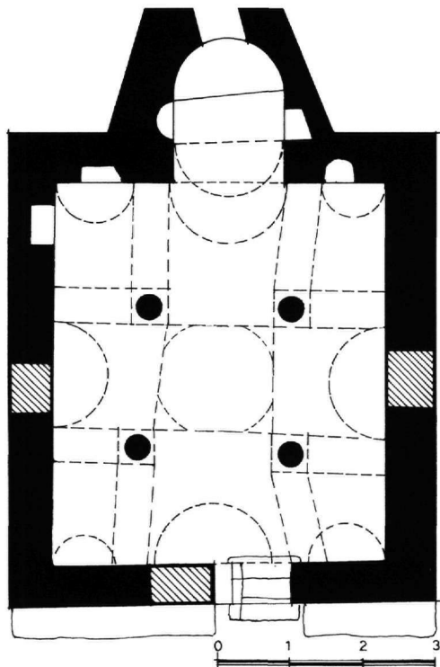
Εικ. 2. Άγιος Αθανάσιος στα Μέγαρα. Κάτοψη του ναού.
