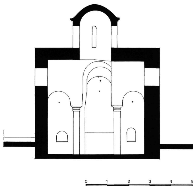
Εικ. 7. Εγκάρσια τομή του ναού.
