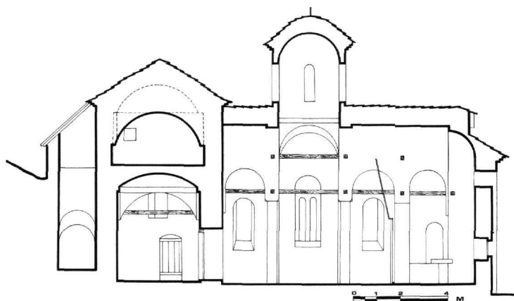
Εἰκ. 3. Ἁγία Τριάδα στή Δέση Τρικάλων. Τομή κατά μήκος.
