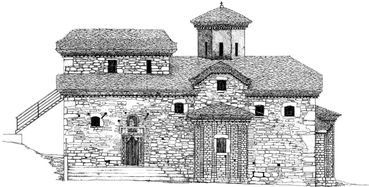
Εἰκ. 12. Ἁγία Παρασκευή στό Νεραΐδοχώρι Τρικάλων. Νότια ὄψη.
