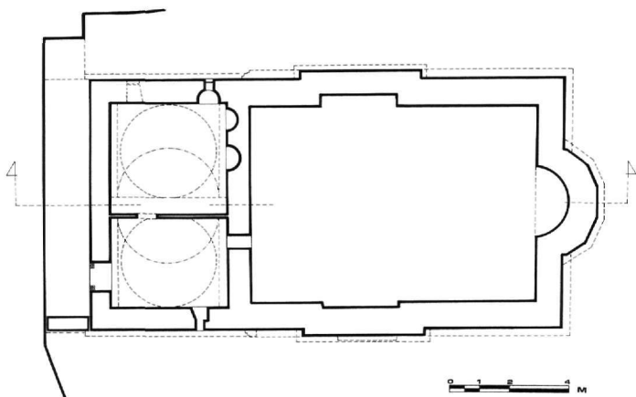
Εικ. 5. Αγία Τριάδα στη Δέση Τρικάλων. Κάτοψη ορόφου.
