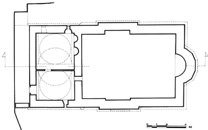
Εἰκ. 5. Αγία Τριάδα στὴ Δέση Τρικιάλων. Κάτοψη ὀρόφου.
