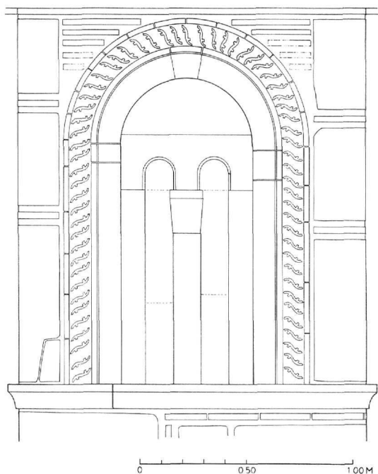
Εικ. 16. Ναός Αγίου Πολυκάρπου. Το παράθυρο της κόγχης του Ιερού. Αναπαράσταση.
