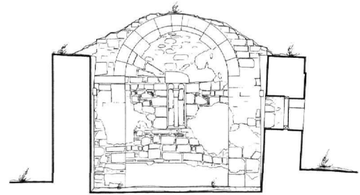
Εικ. 8. Τομή κατά πλάτος.
