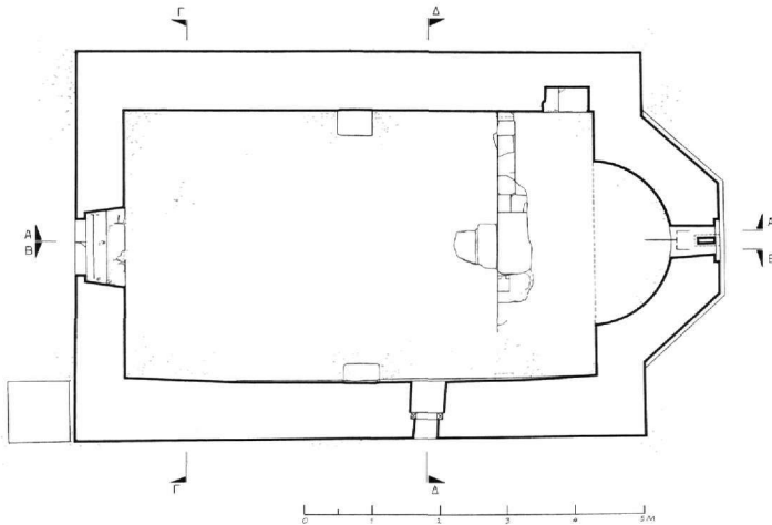
Εικ. 7. Ναός Αγίου Πολυκάρπου. Κάτοψη.
