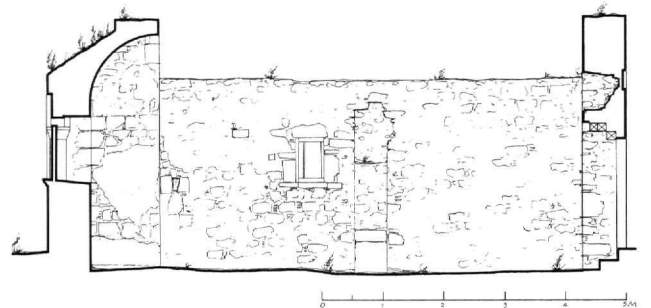
Εικ. 10. Τομή κατά μήκος προς νότον.
