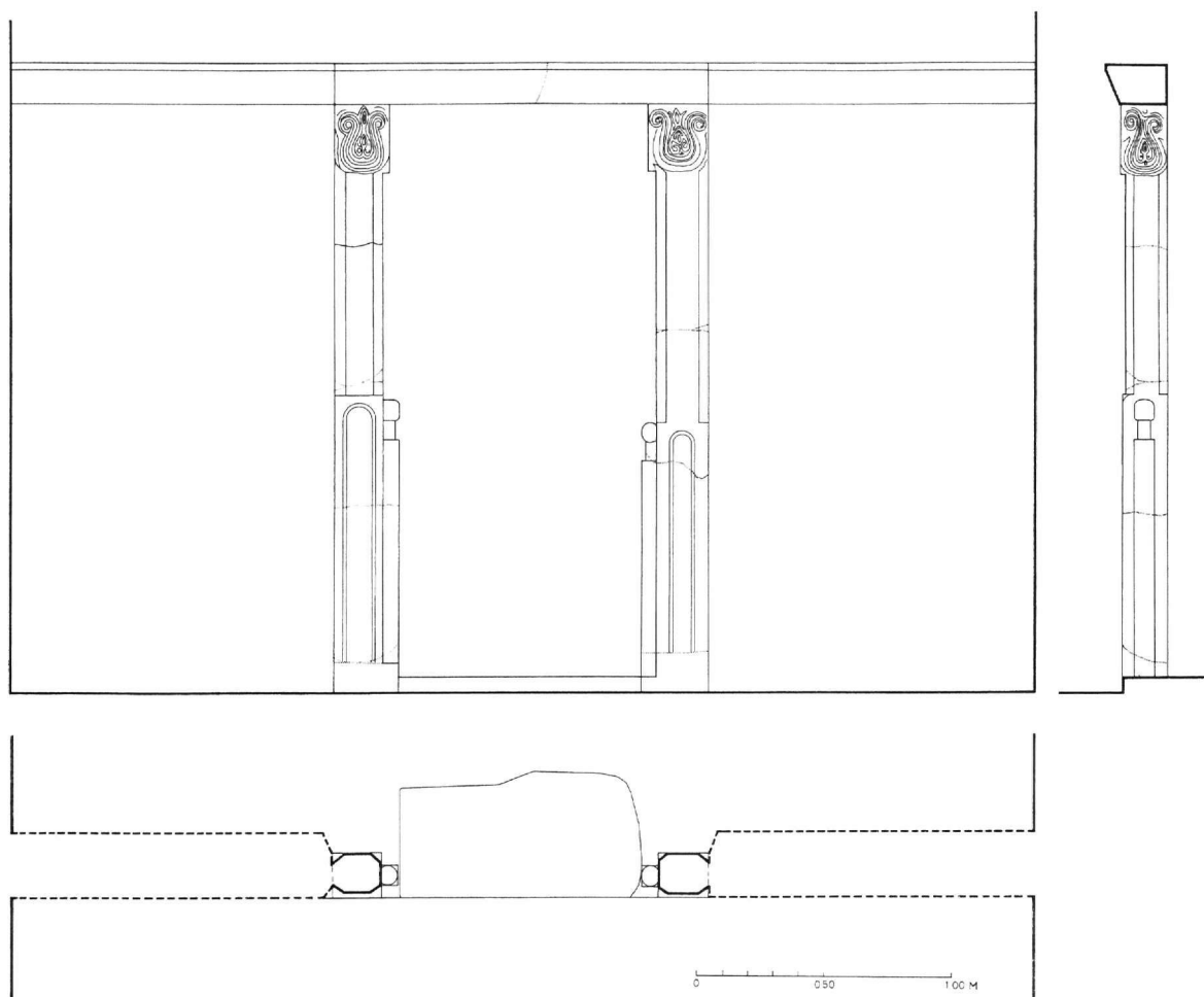
Εικ. 18. Ναός Αγίου Πολυκάρπου. Το τέμπλο. Αναπαράσταση.
