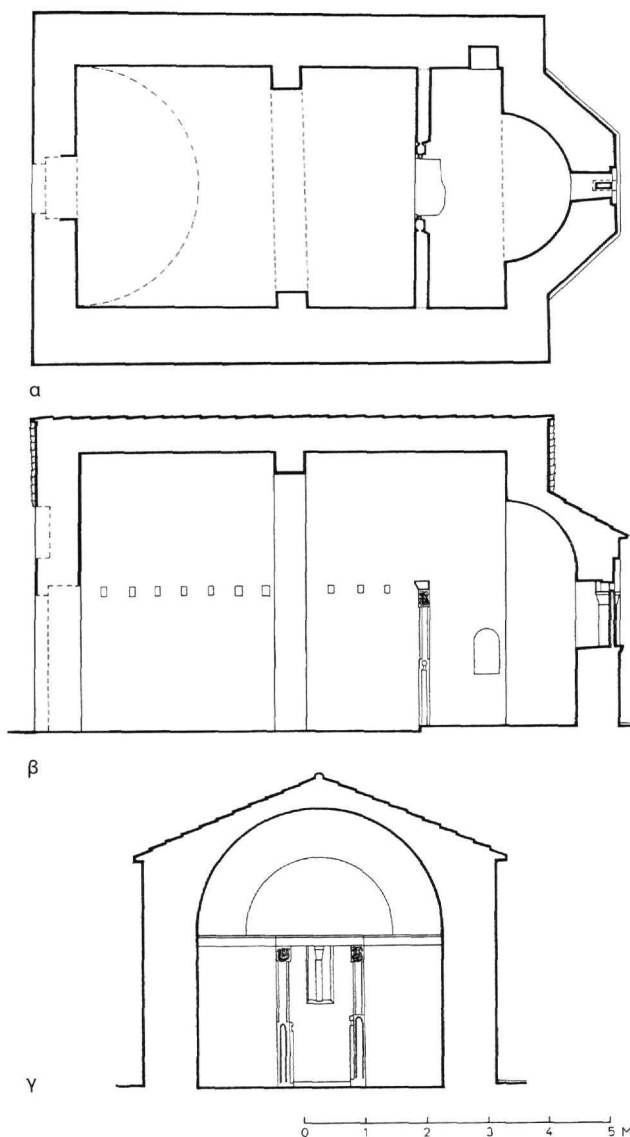
Εικ. 15. Ναός Αγίου Πολυκάρπου. Αναπαράσταση. α. Κάτοψη, β. Τομή κατά μήκος, γ. Τομή κατά πλάτος.
