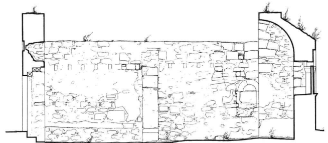
Εικ. 9. Τομή κατά μήκος προς βορράν.
