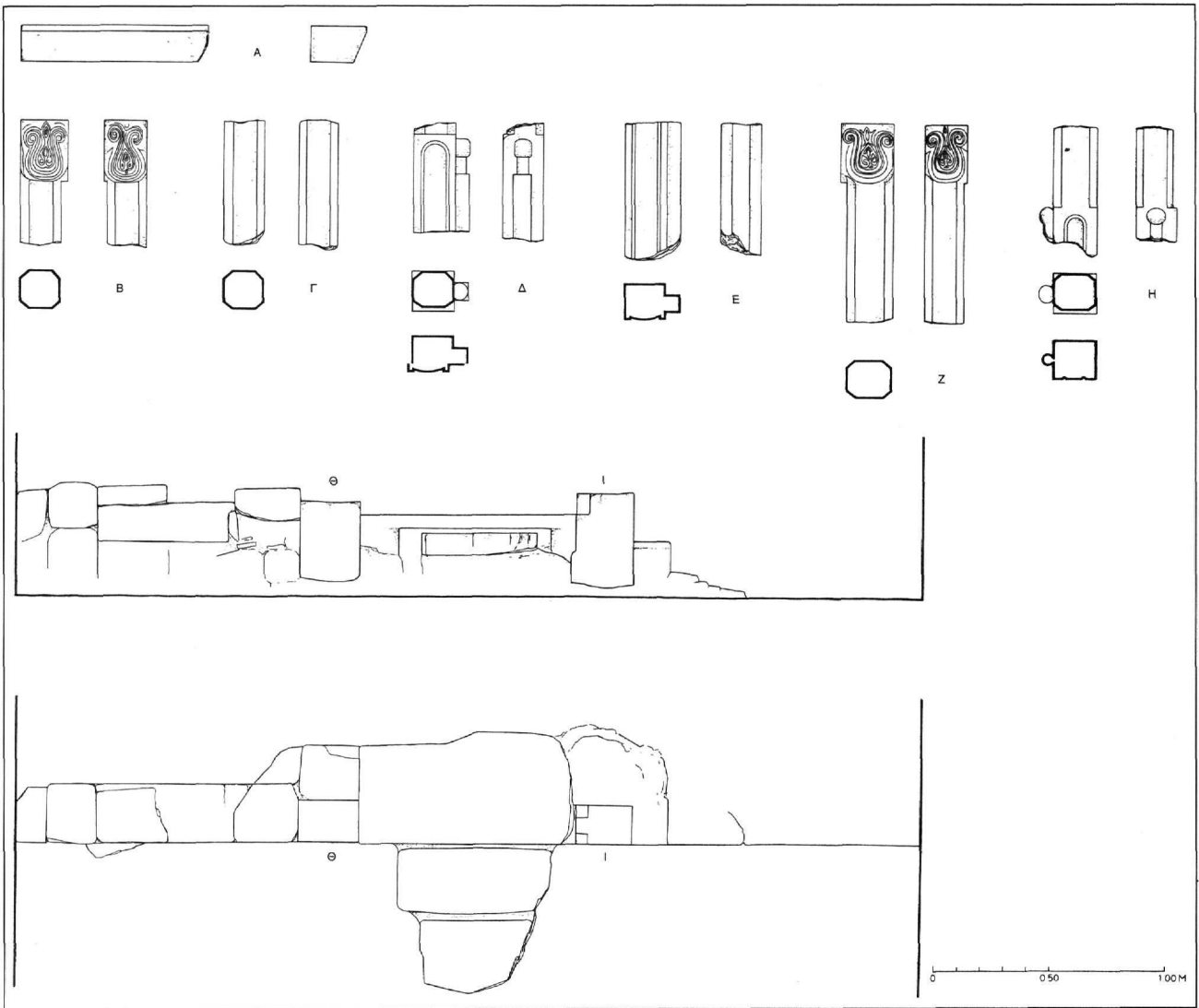
Εικ. 14. Τα λείβανα του τέμπλου.
