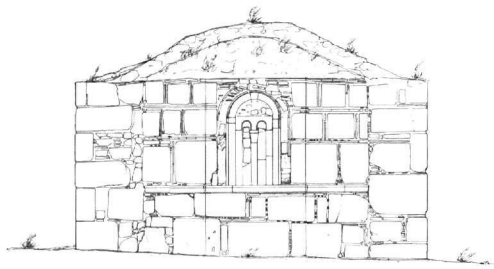
Εικ. 11. Η ανατολική όψη.
