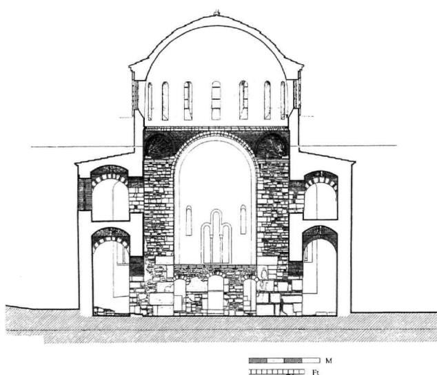
Εικ. 5. Ναός Μεταμορφώσεως του Σωτήρος Χριστιάνων. Τομή κατά πλάτος στον τρούλο από Δ.
