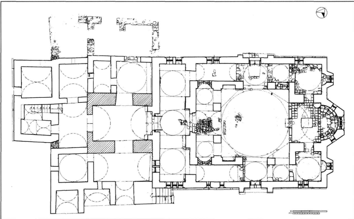
Εικ. 2. Ναός Μεταμορφώσεως του Σωτήρος Χριστιάνων. Κάτοψη κατώτερης στάθμης.
