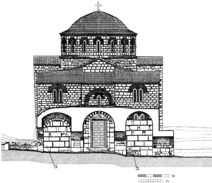
Εικ. 11. Ναός Μεταμορφώσεως του Σωτήρος Χριστιάνων. Τομή κατά πλάτος στο επισκοπέιο.
