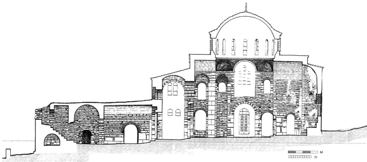
Εικ. 4. Ναός Μεταμορφώσεως του Σωτήρος Χριστιάνων. Τομή κατά μήκος.
