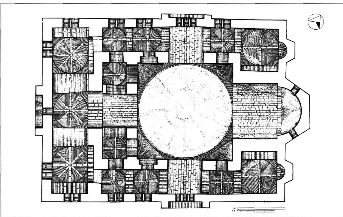
Εικ. 3. Ναός Μεταμορφώσεως του Σωτήρος Χριστιάνων. Ανοψη ανώτερης στάθμης.
