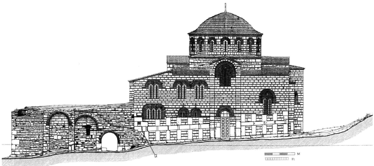
Εικ. 8. Ναός Μεταμορφώσεως του Σωτήρος Χριστιάνων. Νότια πλευρά.
