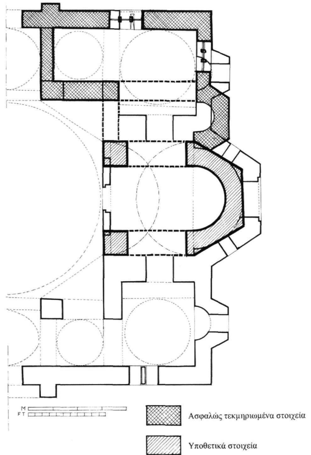
Εικ. 20. Ναός Μεταμορφώσεως του Σωτήρος Χριστιάνων. Γραφική αποκατάσταση της 2ης φάσης βασισμένη στα ευρήματα των ερευνητικών εργασιών.
