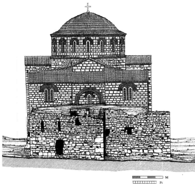
Εικ. 10. Ναός Μεταμορφώσεως του Σωτήρος Χριστιάνων. Δυτική πλευρά.
