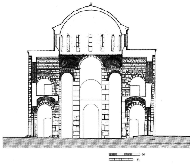
Εικ. 6. Ναός Μεταμορφώσεως του Σωτήρος Χριστιάνων. Τομή κατά πλάτος στον τρούλο από Α.
