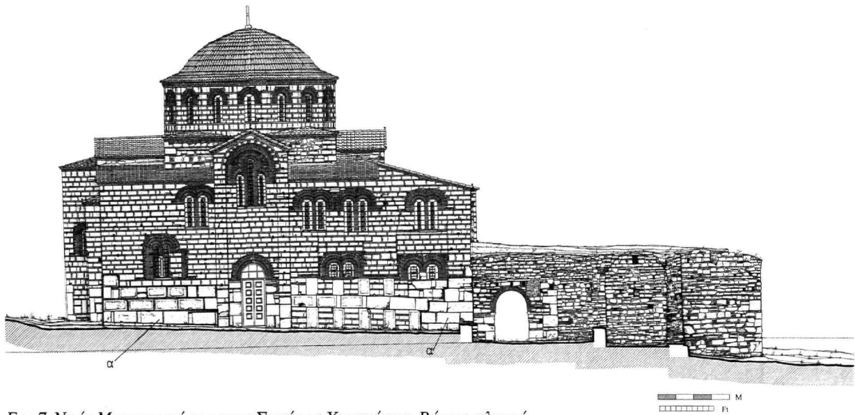
Εικ. 7. Ναός Μεταμορφώσεως του Σωτήρος Χριστιάνων. Βόρεια πλευρά.
