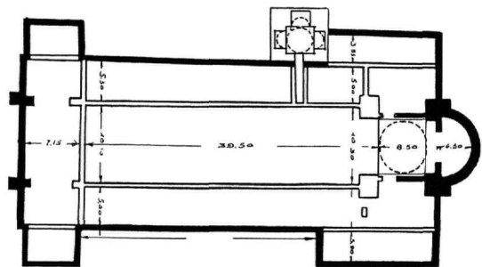
Εικ. 2. Κάτοψη της βασιλικής του Ιλισού.
