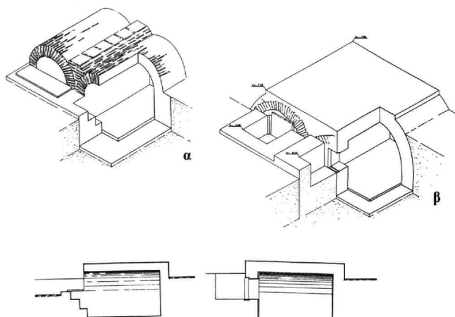
Εικ. 4. Αξονομετρικό και τομή καμαρωτού τάφου: α με οριζόντια είσοδο και β με κάθοδο.
