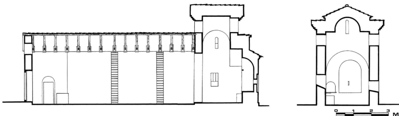
Εικ. 3-4. Οί Ταξiάρχes στο Έλάφι Καλαμπάκας. Τομή κατά πλάτος και εγκάρσια.
