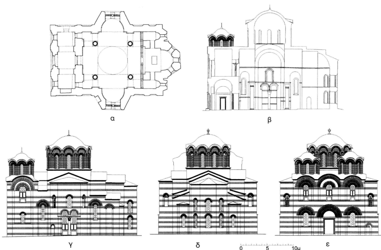
Εικ. 3. Καθολικό μονής Βατοπεδίου. Αναπαράσταση: α. Κάτοψη, β. Τομή κατά μήκος, γ. Νότια όψη, δ. Ανατολική όψη, ε. Δυτική όψη.
