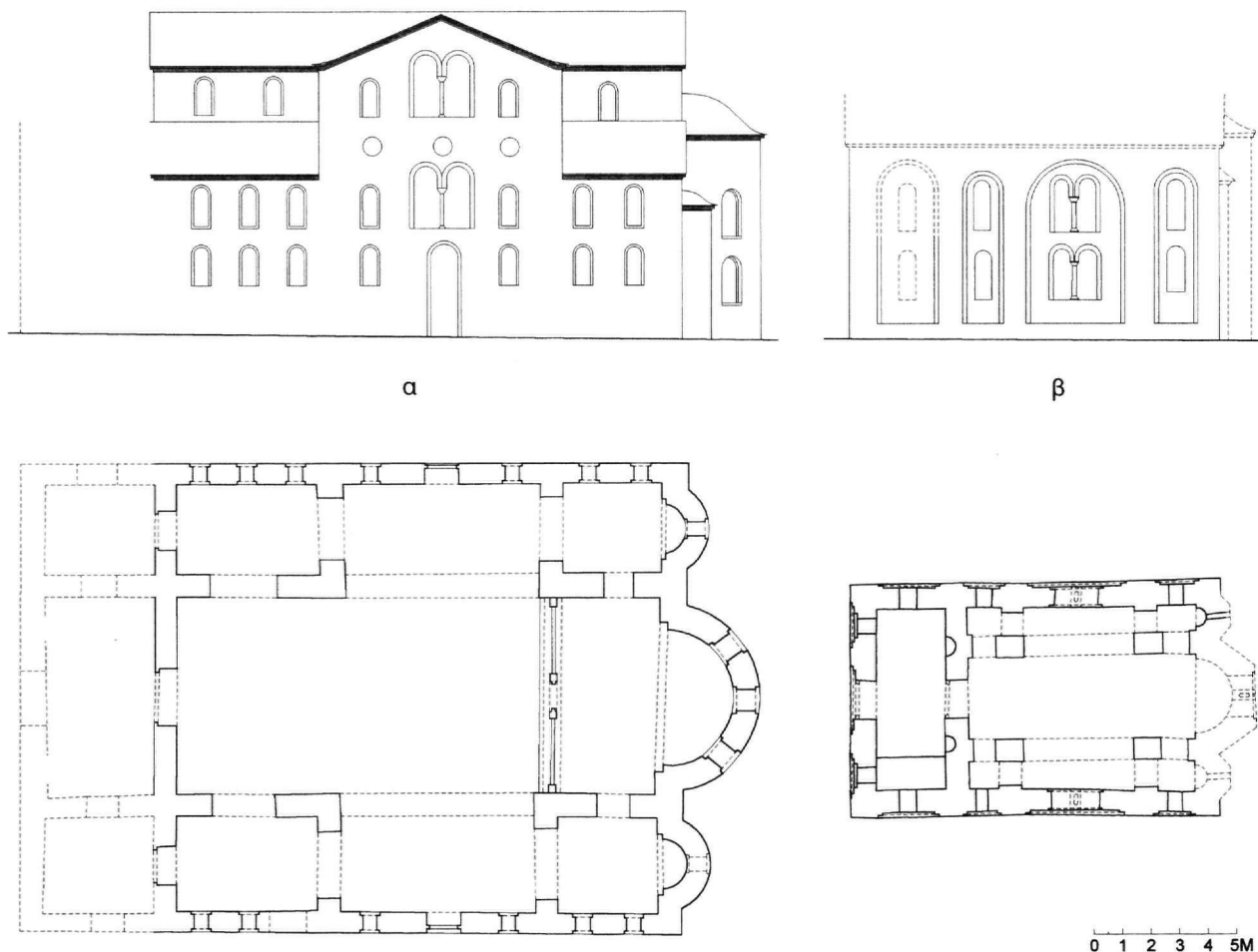
Εικ. 9. α. Ναός Πρωτάτου Καρυνών. Αναπαράσταση: Κάτοψη και νότια όψη (βάσει σχεδίου Π. Φουντά). β. Ναός Κελλίον Ραβδούχον Καρυνών. Αναπαράσταση: Κάτοψη και νότια όψη.
