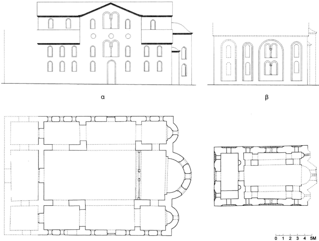
Εικ. 9. α. Ναός Πρωτάτου Καρών. Αναπαράσταση: Κάτοψη και νότια όψη (βάσει σχεδίου Π. Φουντά). β. Ναός Κελλίου Ραβδούχων Καρών. Αναπαράσταση: Κάτοψη και νότια όψη.
