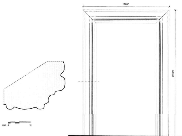
Εικ. 5. Όψη θυρώματος της Ωραίας Πύλης και εμφανές τμήμα της διατομής του.
