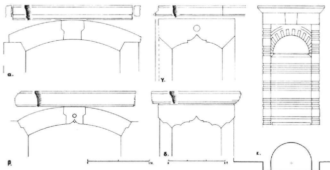
Εἰκ. 7. Καθολικό μονῆς Ἁγίου Δημητρίου Στομίον. Λεπτομέρειες: α) Τόξο τῆς εἰσόδου στόν κυρίως ναό. β) Τόξο τῆς εἰσόδου τῆς λιτῆς. γ) Τόξο τῆς βορείας εἰσόδου τῆς λιτῆς. δ) Τόξο τῆς νοτίας εἰσόδου τῆς λιτῆς. ε) Κάτοψη καί τομή τῆς παραστάδος μέ κογχάριο στήν λιτή.
