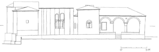
Εἰκ. 4. Καθολικό μονής Ἁγίου Δημητρίου Στομίου. Σχηματική βόρεια πρόσοψη στήν υπάρχουσα κατάσταση.
