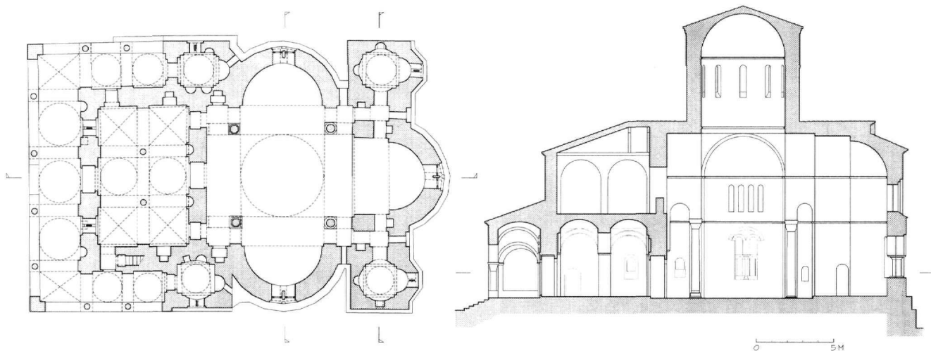
Εἰκ. 12. Καθολικό μονῆς Ἁγίου Δημητρίου Στομίον. Κάτοψη καί κατά μήκος τομή σέ ἀποκατάσταση.
