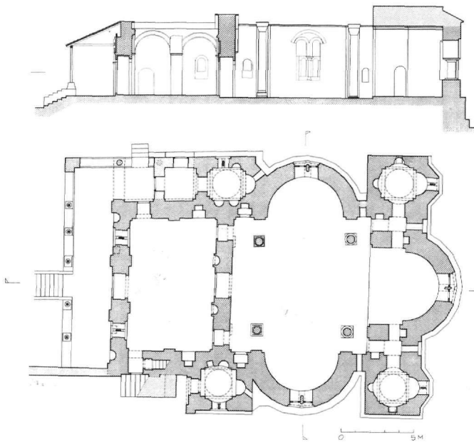
Εικ. 3. Καθολικό μονής Ἁγίου Δημητρίου Στομίου. Κάτοψη καὶ κατά μήκος τομή στὴν ὑπάρχουσα κατάσταση.
