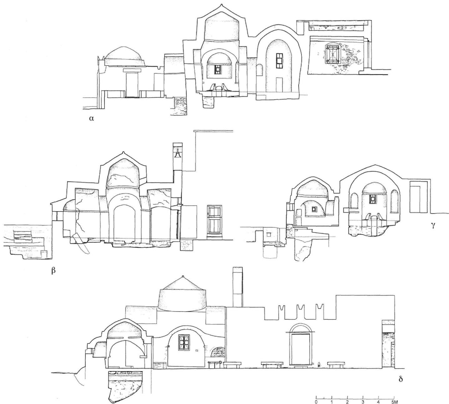
Εικ. 4. Συγκρότημα Αγίων Αναργύρων. α: Τομή ΑΑ, β: Τομή ΒΒ, γ: Τομή ΓΓ, δ: Τομή ΔΔ.
