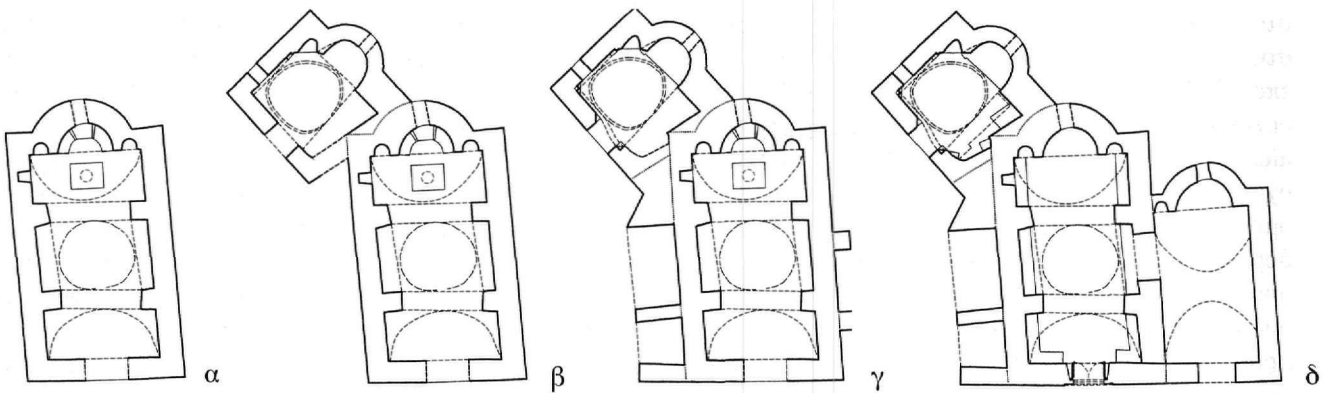
Εικ. 7. Συγκροτήμα Αγίων Αναργύρων. Οικοδομικές φάσεις - Αναπαραστάσεις.
