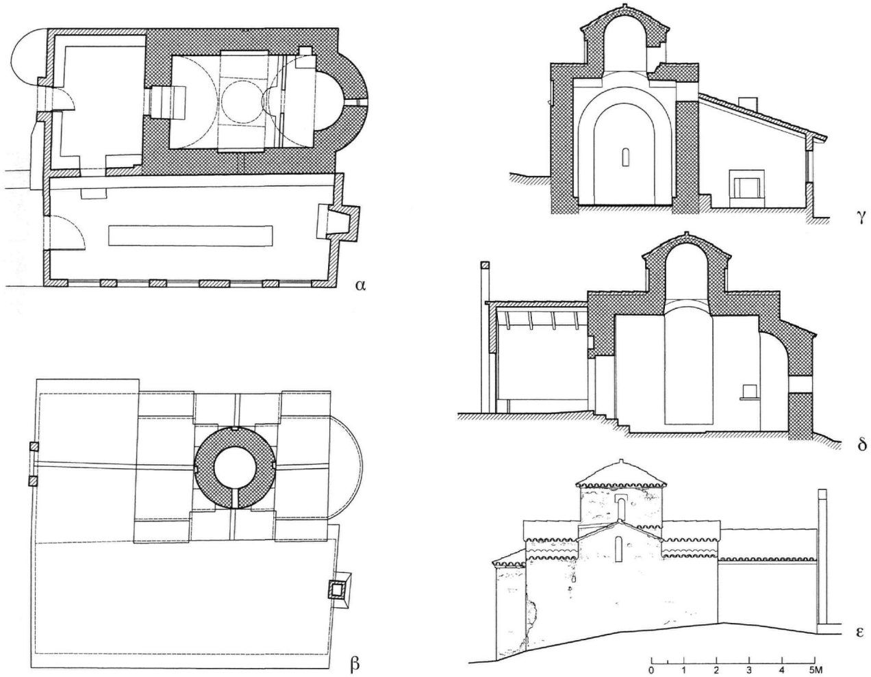
Εικ. 2. Υπαπαντή Σοφικού: α. Κάτοψη, β. Κάτοψη της στέγης, γ. Τομή κατά πλάτος, δ. Τομή κατά μήκος προς Β, ε. Βόρεια όψη.
