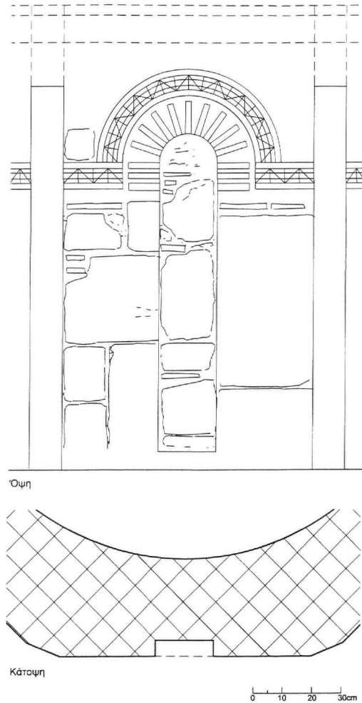
Εικ. 8. Άγιος Αντώνιος στην Τούλα Σοφικού. Νοτιοανατολική πλευρά του τυμπάνου του τρούλου. Γραφική αποκατάσταση (όψη και κάτοψη).
