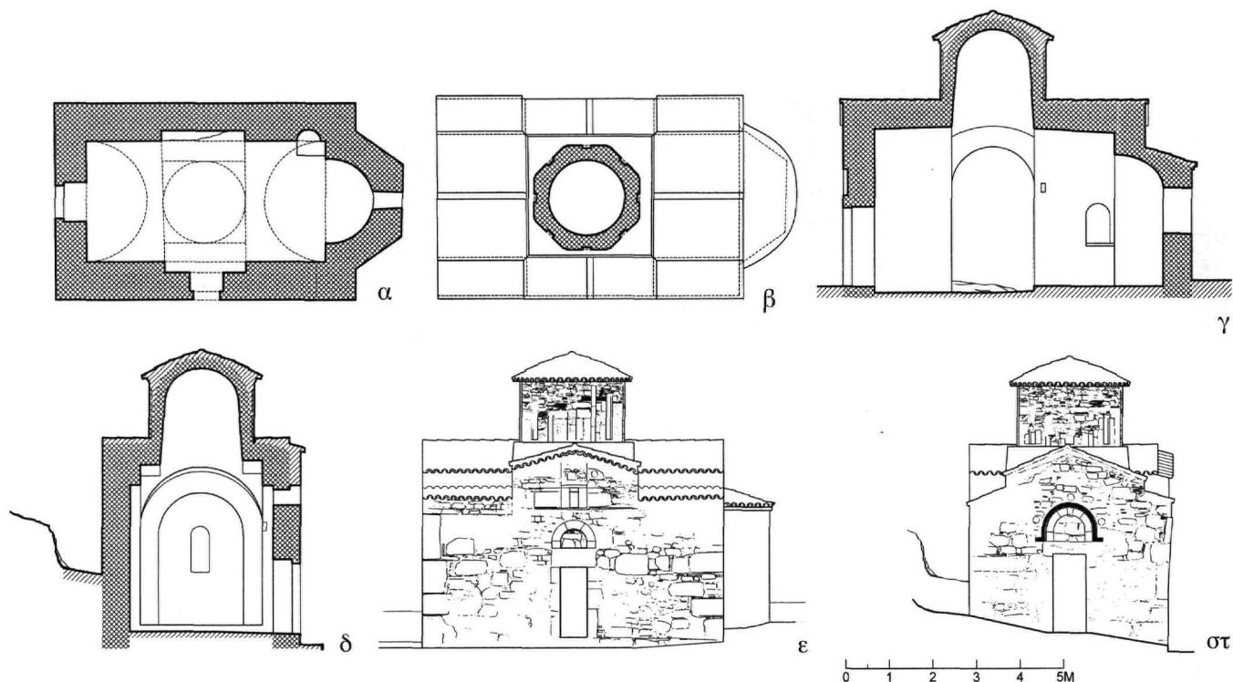
Εικ. 6. Άγιος Αντώνιος στην Τούρλα Σοφικού. α. Κάτοψη, β. Κάτοψη της στέγης, γ. Τομή κατά μήκος προς Β., δ. Τομή κατά πλάτος, ε. Νότια όψη, στ. Δυτική όψη.
