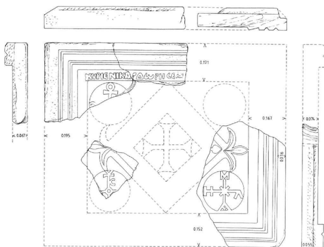
Εικ. 14. Σχέδιο αποκατάστασης θωρακίων τέμπλου (τμήματα E139, E218, E141, E142).
