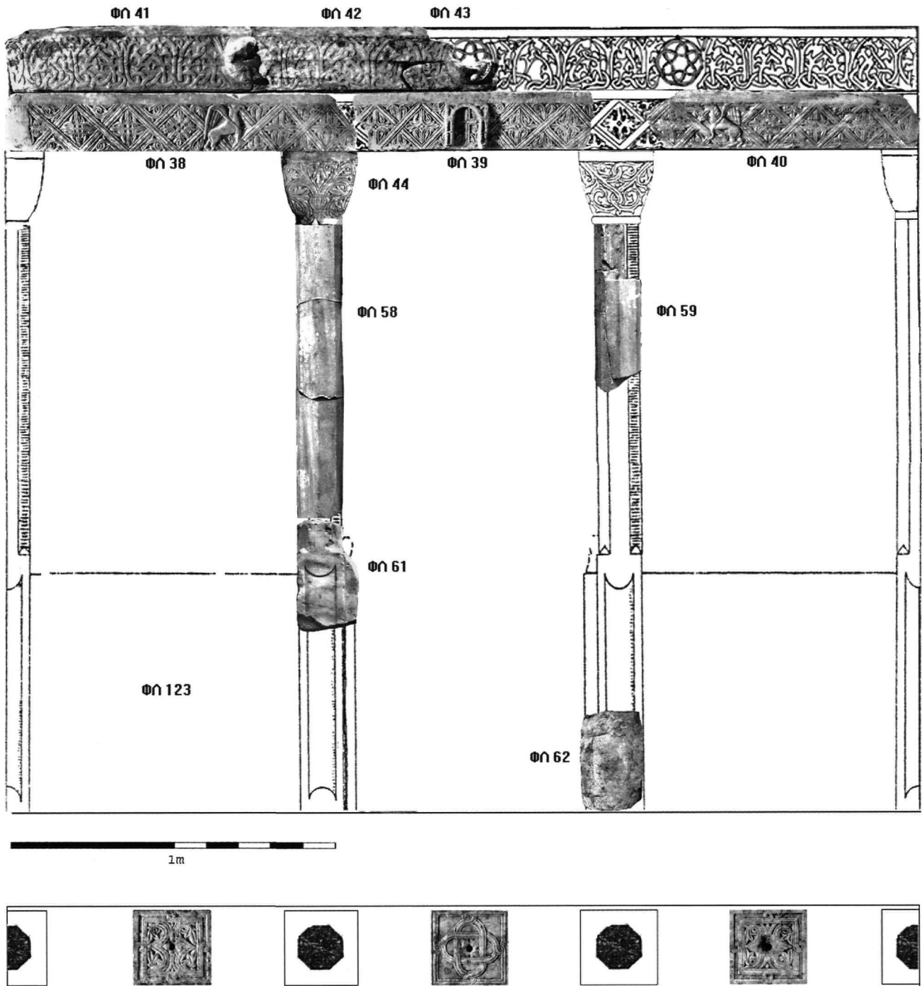
Εικ. 1. Ταξιάρχης Λοκρίδας. Αποκατάσταση τέμπλου ιερού βήματος.
