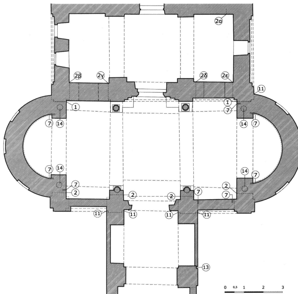
Εικ. 3. Κάτοψη του εξωνάρθηκα και του εσωνάρθηκα: 1. Οικοδομικός αρμός εσωνάρθηκα-εξωνάρθηκα, 2. Οικοδομικός αρμός, 7. Τηχη ορθομαρμάρωσης, 11. Αρχικό επίχρισμα με απομίμηση ισόδομου, 13. Ρόδινο επίχρισμα, 14. Πιθανή θέση κιώνων.
