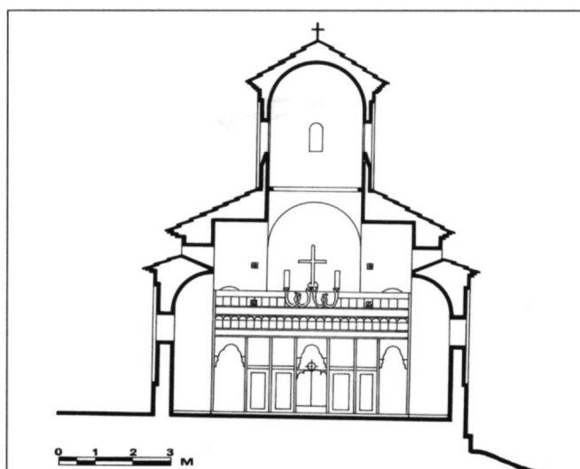
Εικ. 5. Καθολικό της μονής Κλεινοῦ. Τομή κατά πλάτος.
